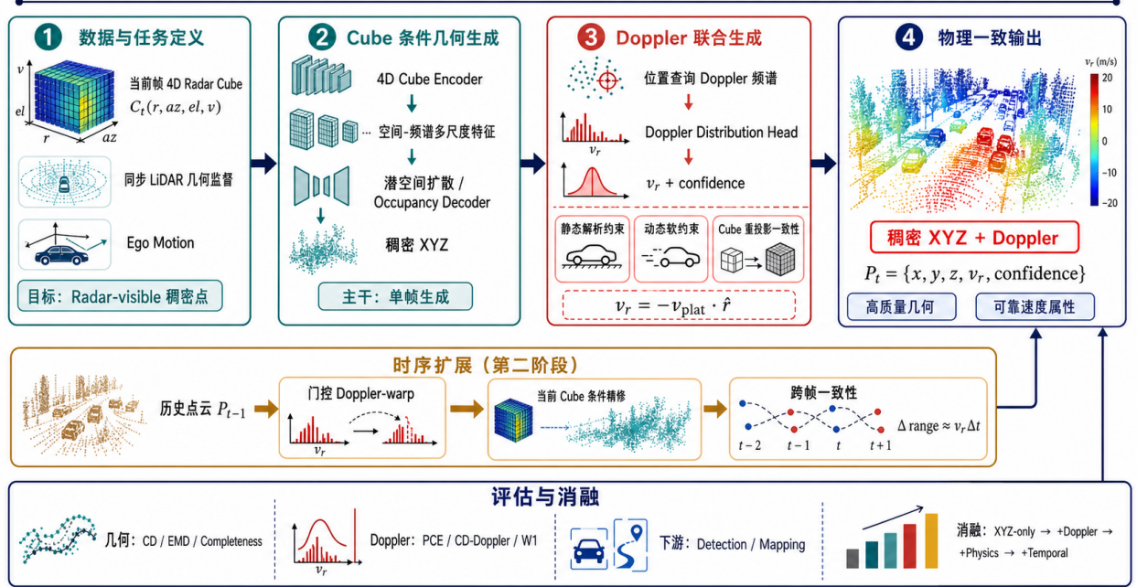
图 1: 目标系统技术路线。当前已验证的是数据协议与单帧几何诊断; 图中的 Doppler 联合生成、Cube 重投影闭环和时序扩展仍受几何父模型门控, 本图不表示这些下游模块已经通过实验。
