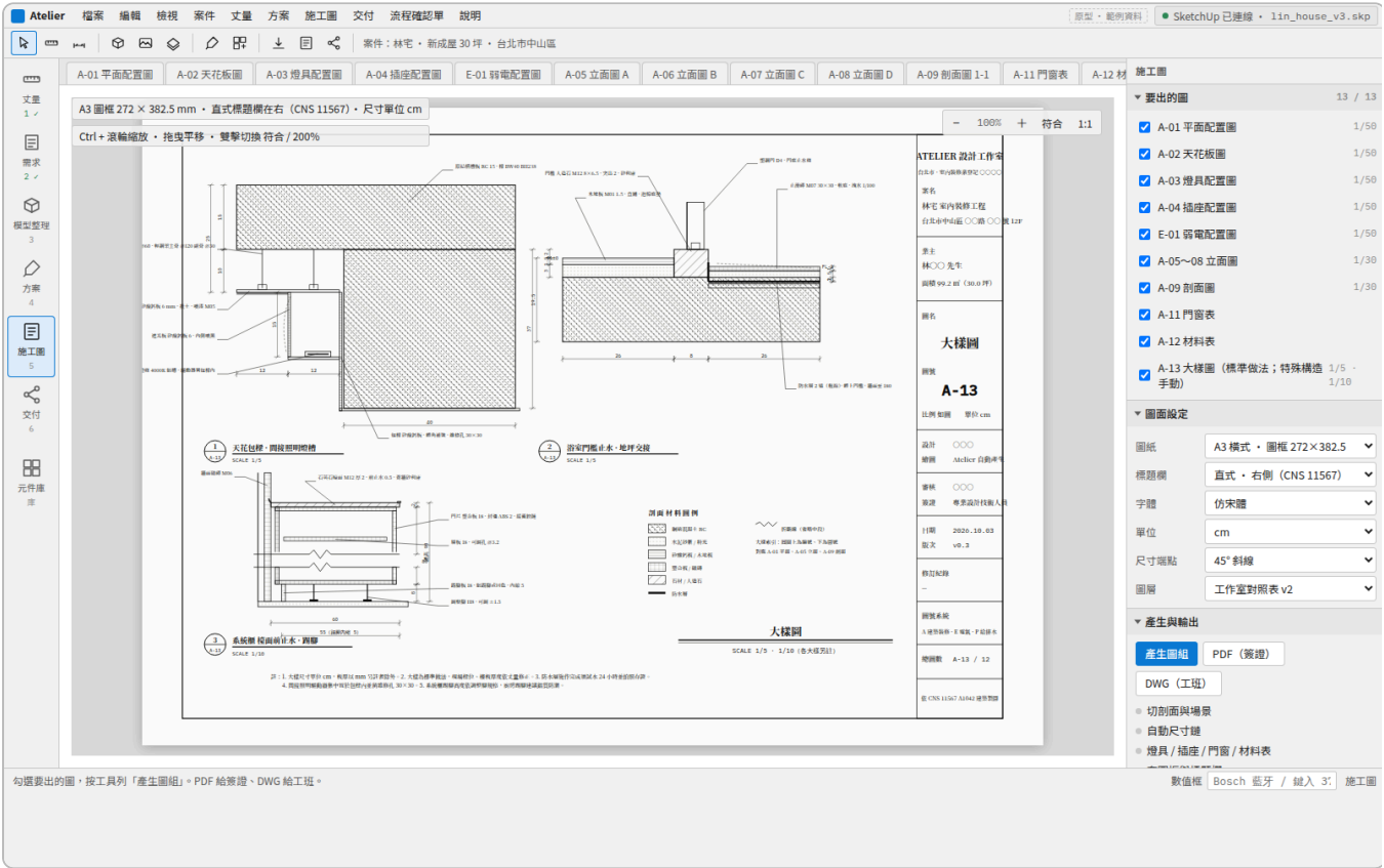
A-13 大樣圖：天花燈槽、浴室門檻止水、系統櫃檯面與踢腳三個標準大樣，1/5 與 1/10。標準大樣由範本自動帶入，特殊構造仍由設計師手畫。
