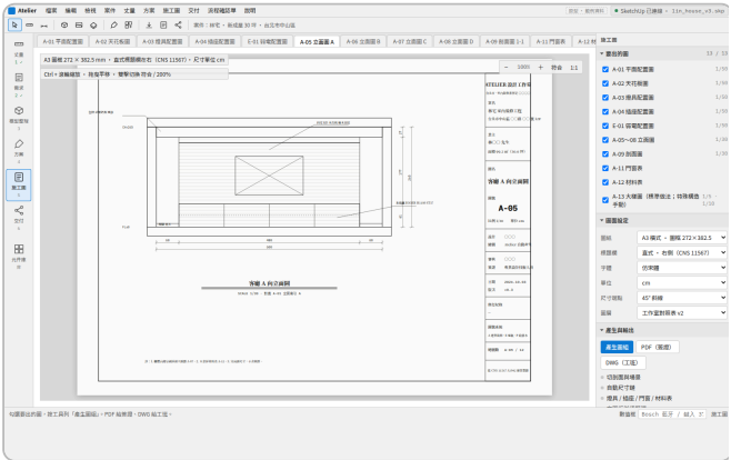
A-05 客廳立面圖 1/30：剖到的樓板斜線、櫃體分割、材料引線、尺寸鍵。
