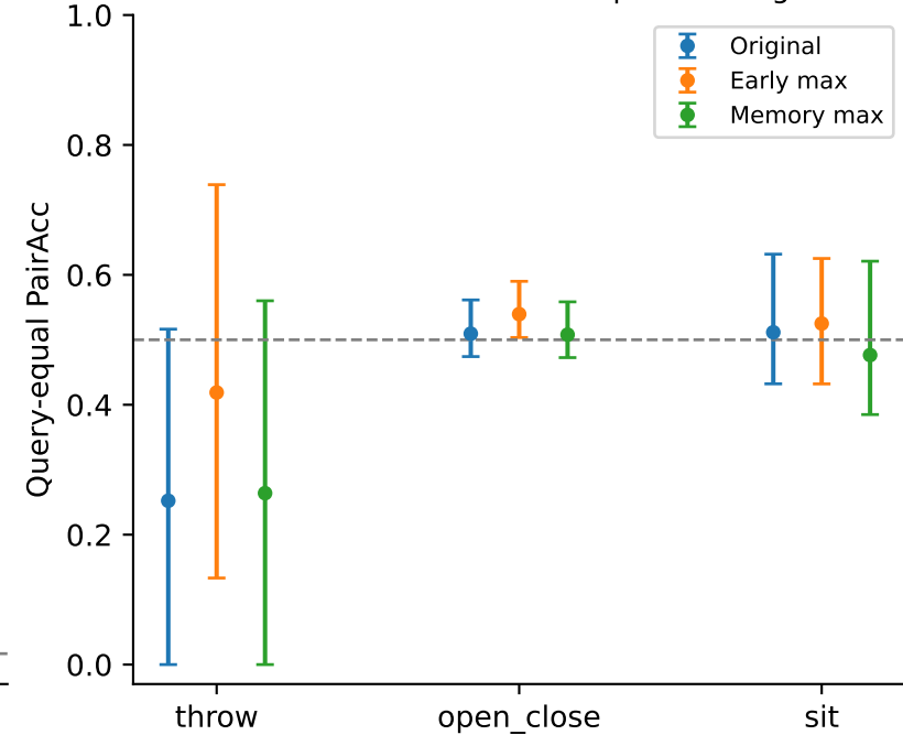
Same actual text: visual pair ranking
