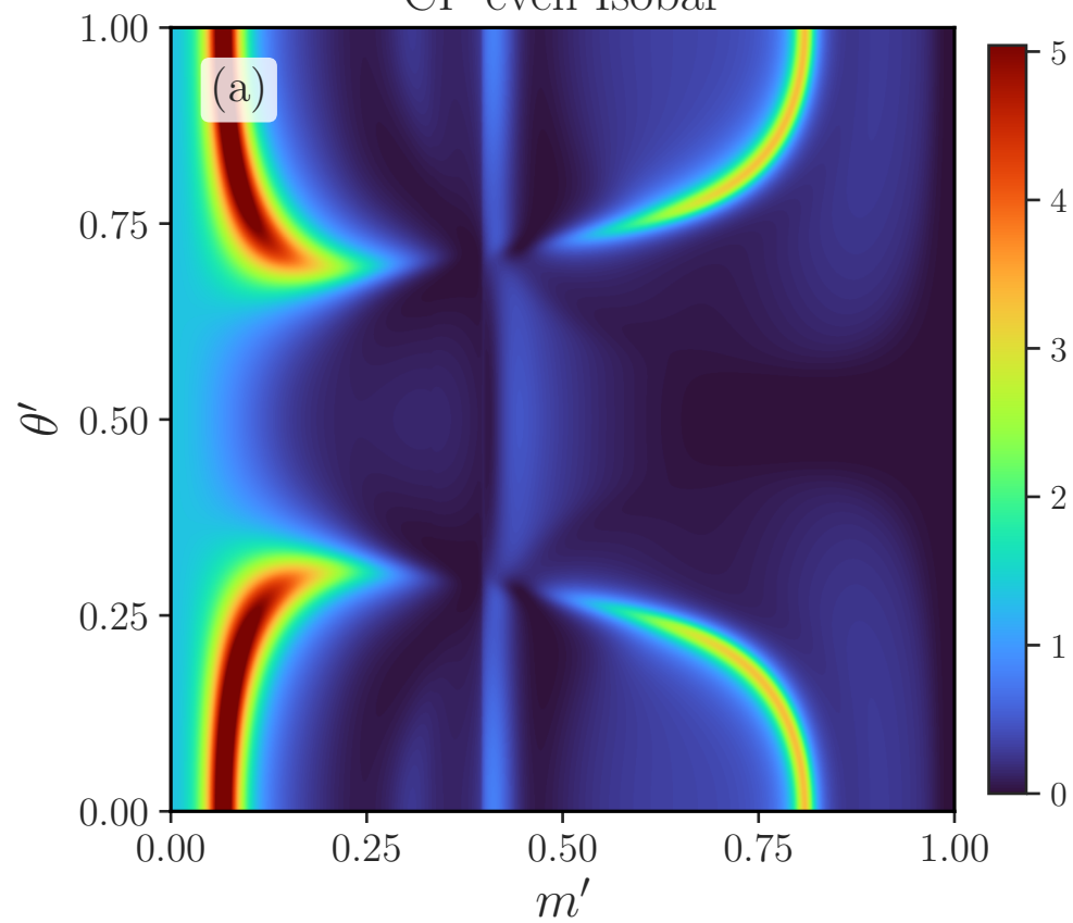
CP-even Isobar
