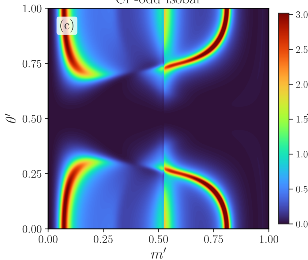
CP-odd Isobar
