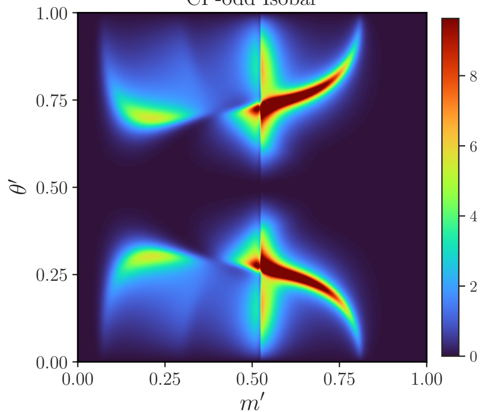
CP-odd Isobar
