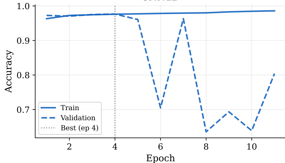
ECAPA-VAD
