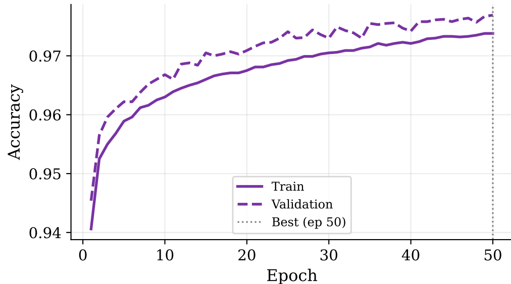
Transformer-VAD
