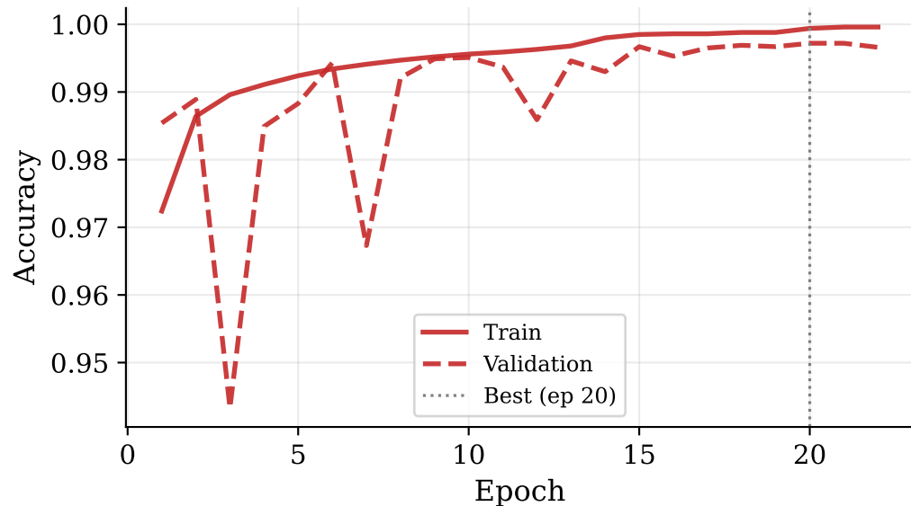
ECAPA-VAD
