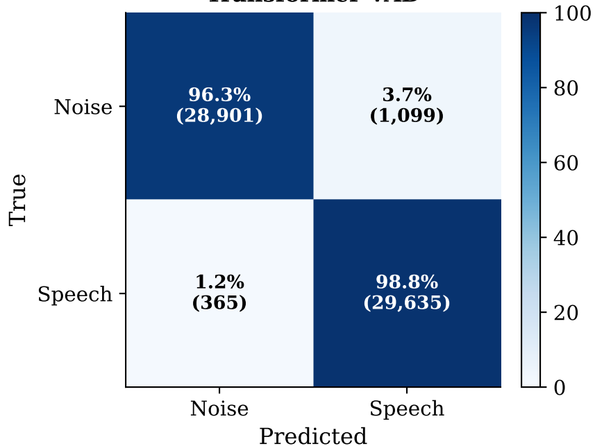
Transformer-VAD
