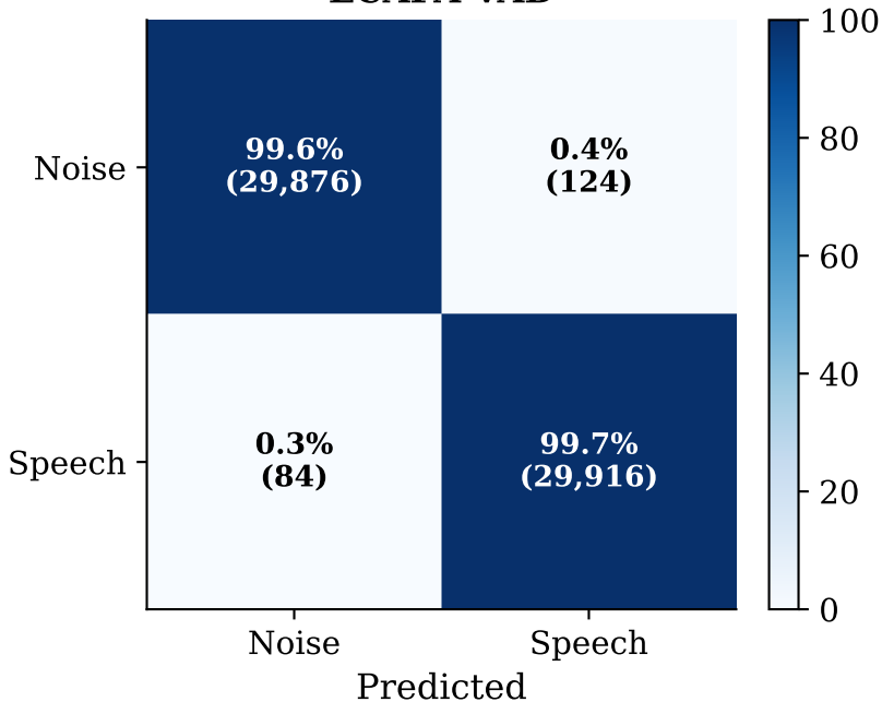
ECAPA-VAD
