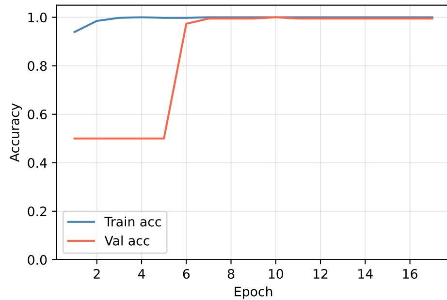
CNN1D
