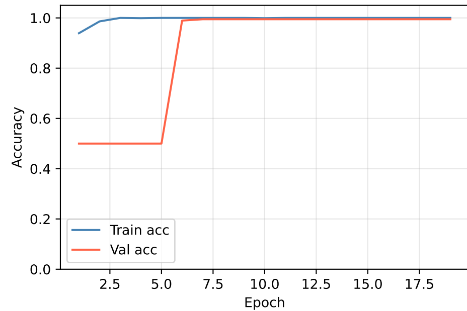
ECAPAVAD
