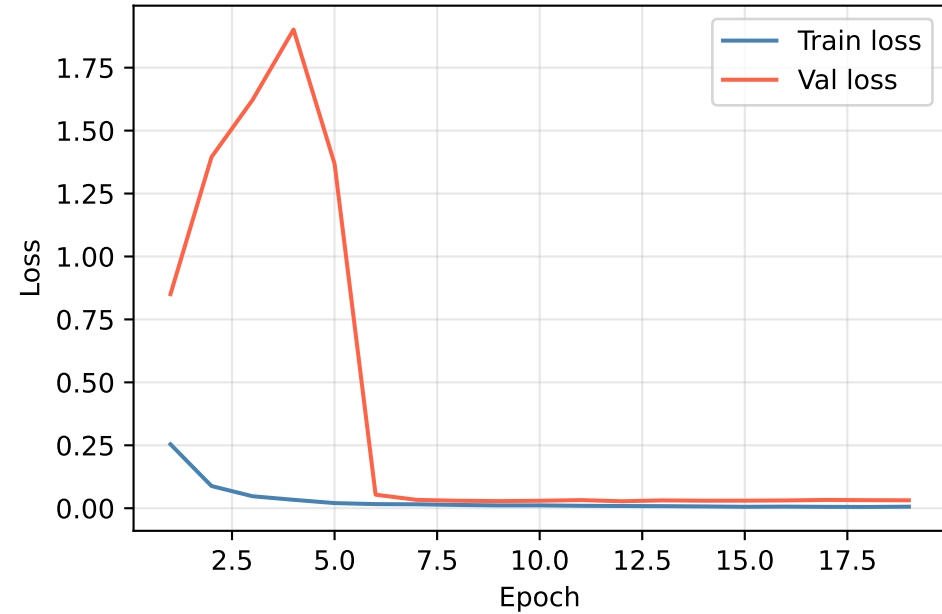
ECAPAVAD
