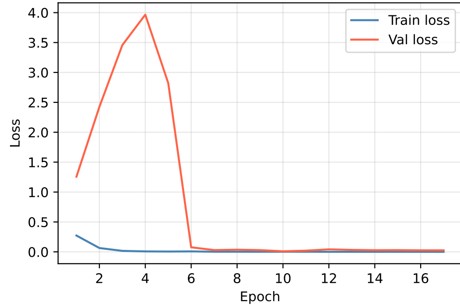
CNN1D
