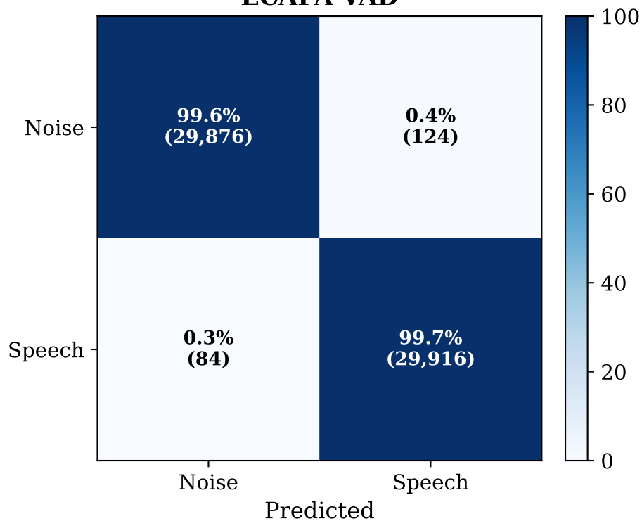
ECAPA-VAD
