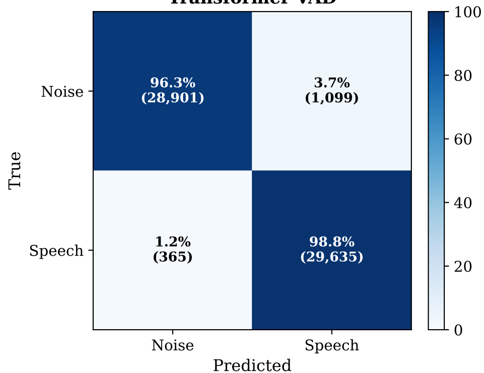
Transformer-VAD
