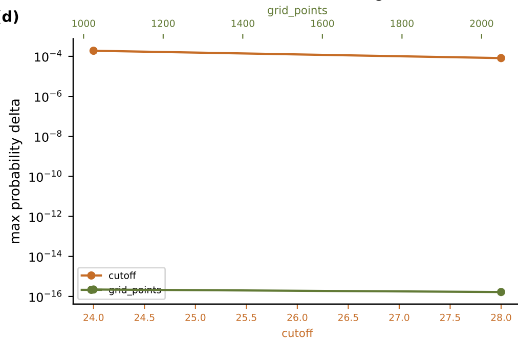
(d) Numerical-refinement convergence (R47)
