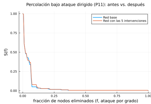
Figura 7: Curva de percolación bajo ataque dirigido por grado: red base (azul) frente a red con las cinco intervenciones (naranja). La mejora es real pero modesta —coherente con cinco enlaces sobre 209— y visible sobre todo en el tramo f \in [0,05; 0,20] .
