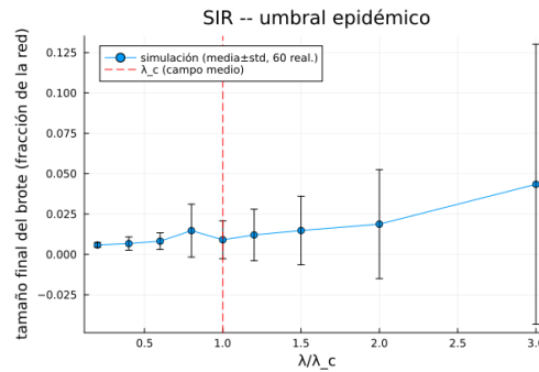
Figura 6: Tamaño final del brote SIR (fracción de la red) frente a \lambda/\lambda_c , con media \pm desviación estándar sobre 60 realizaciones por punto. La línea vertical discontinua marca el umbral de campo medio \lambda_c = 0,1861 .
