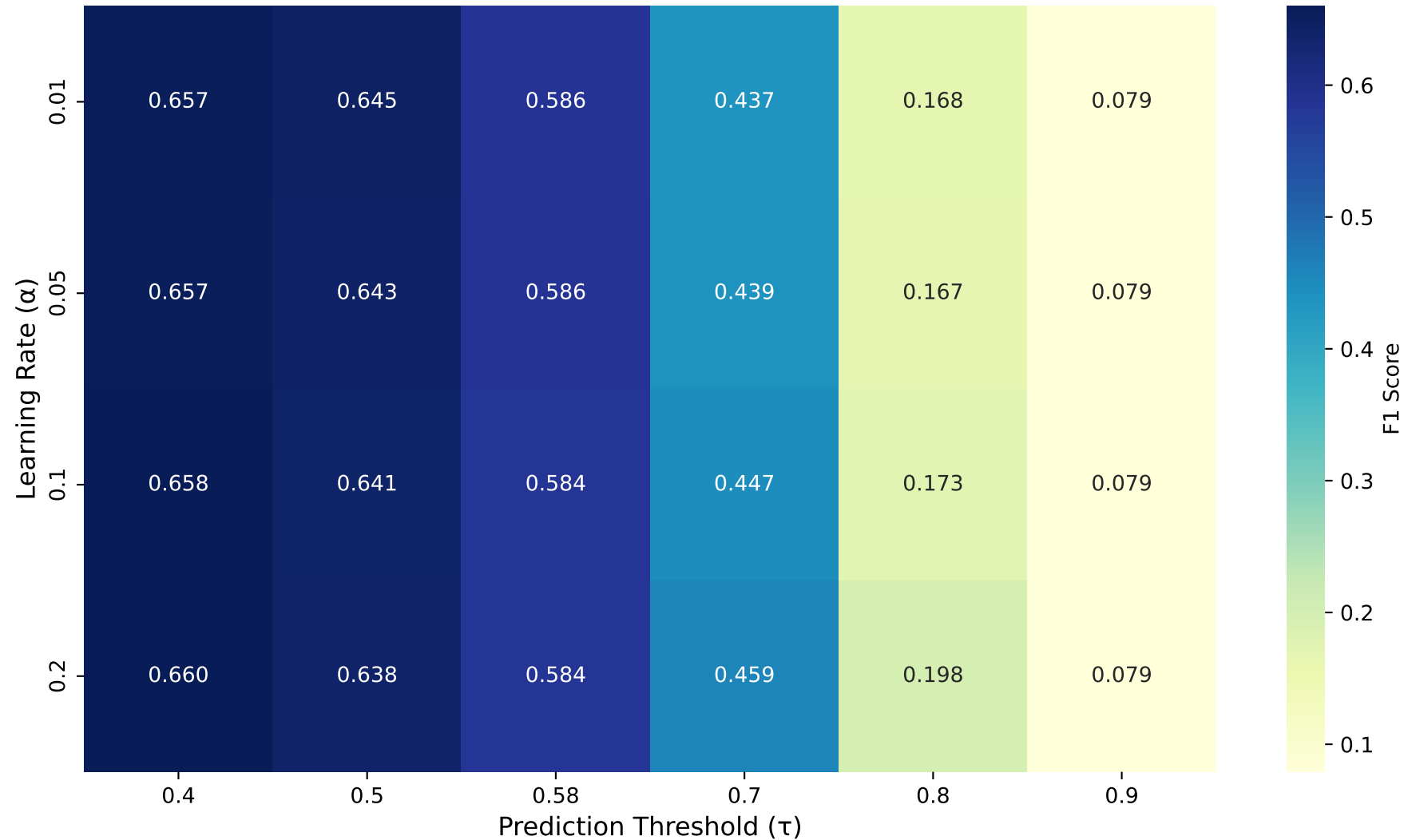
Hyperparameter Sensitivity: F1 Score
