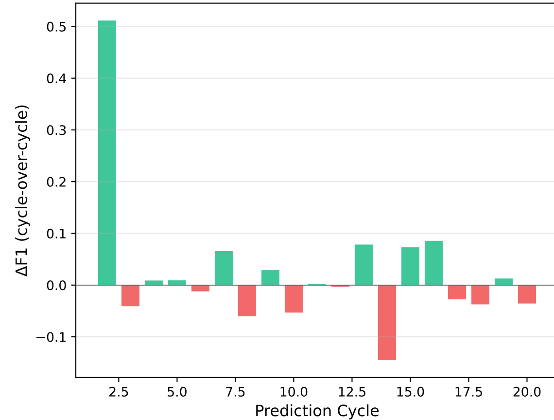
F1 Convergence Rate
