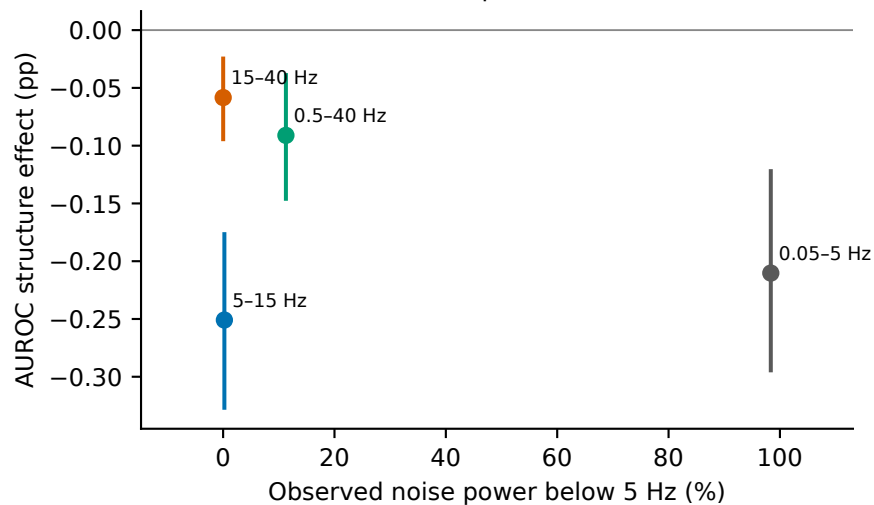
TCN | 10 dB
