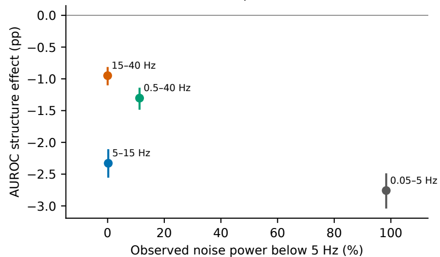
TCN | 0 dB
