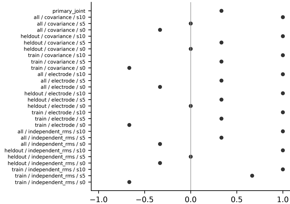
TCN | Kendall
