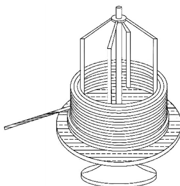
图 E.1 盘卷放线架
