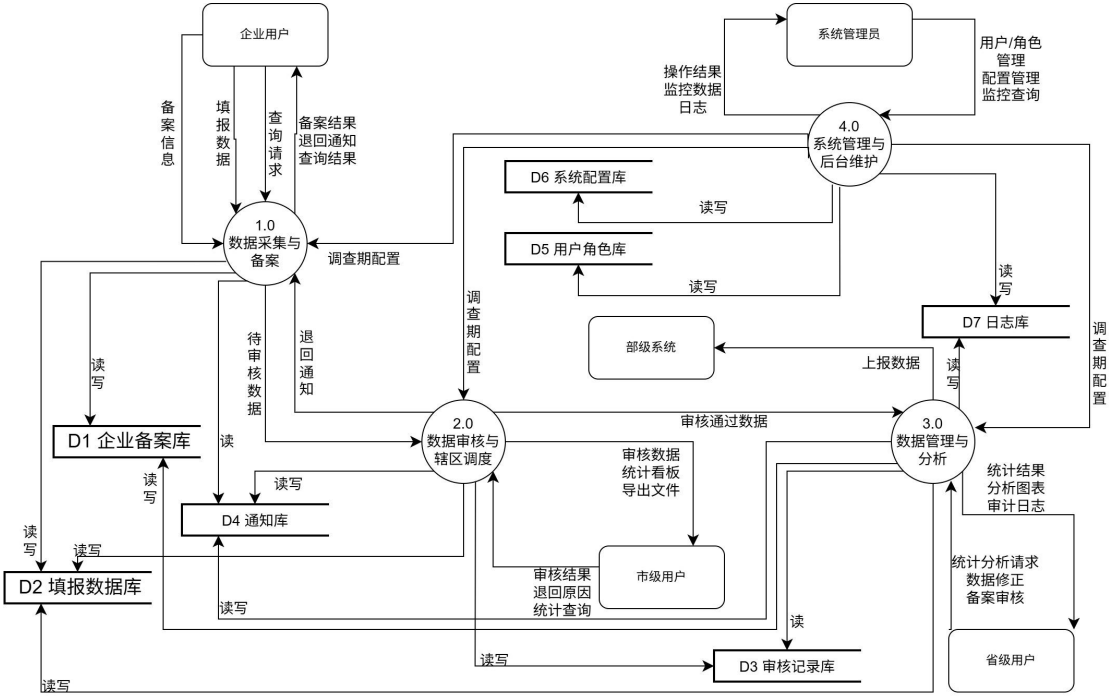
B-5-2 零层图
