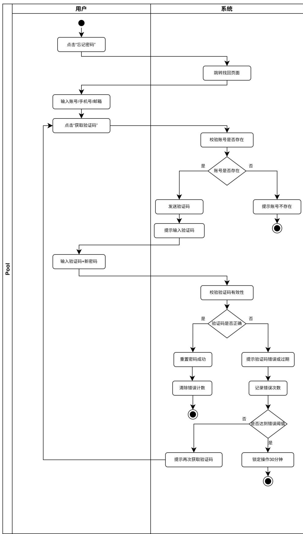
图 B-2-4 账户密码找回与重置活动图
