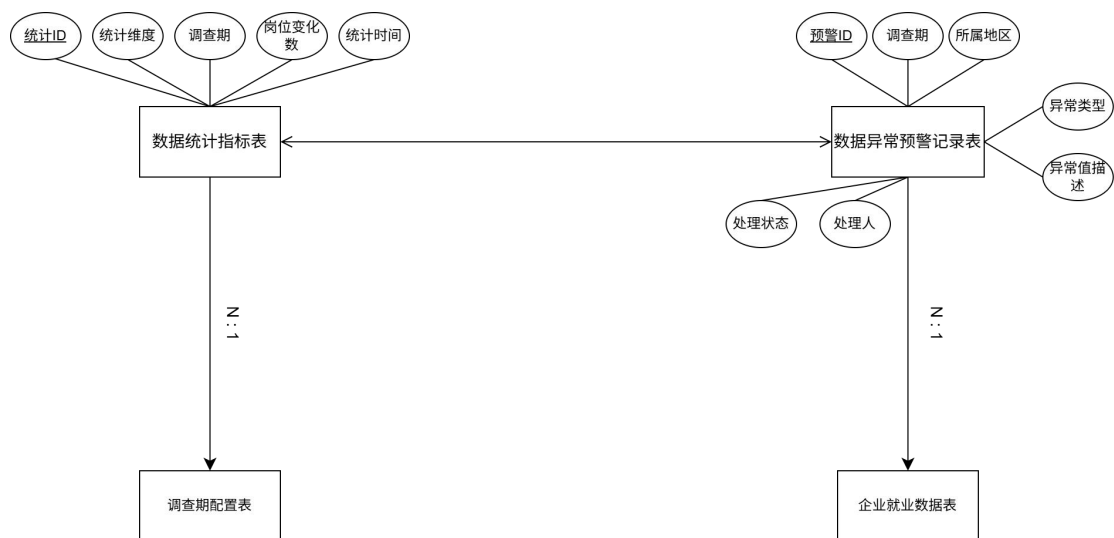
图 B-1-3 省级端：数据管理与分析子系统的 E-R 图
