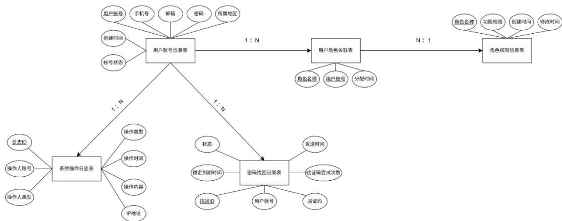
图 B-1-4 省级端：系统管理与后台维护子系统的 E-R 图
