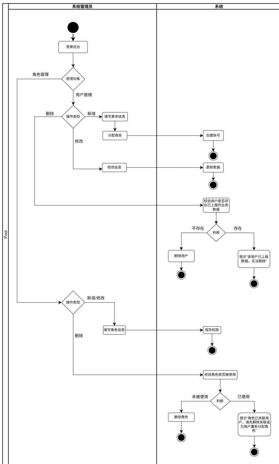
图 B-2-5 系统管理员用户与角色管理活动图
