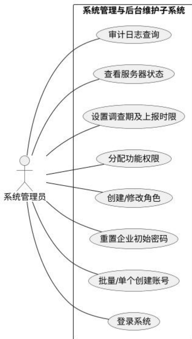
图 B-3-5 省级端：系统管理与后台维护子系统用例图
