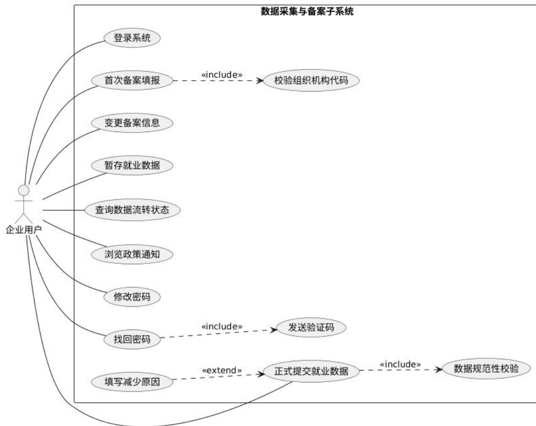
图 B-3-2 企业端：数据采集与备案子系统用例图
