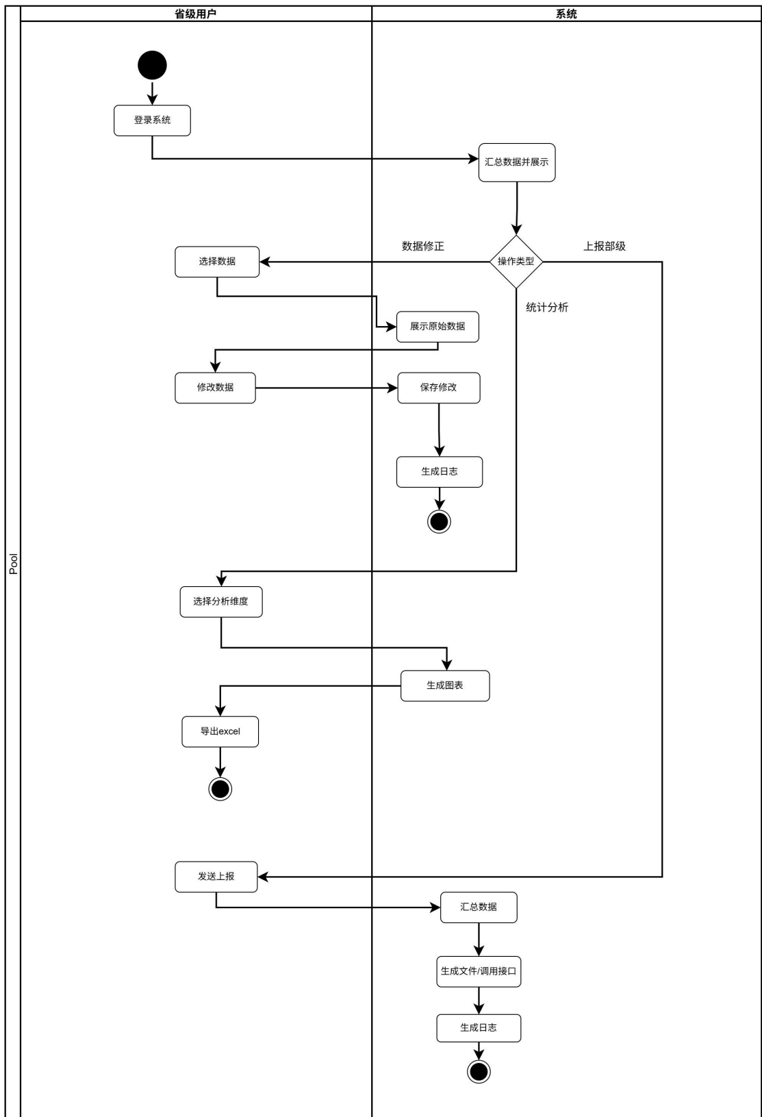
图 B-2-6 省级数据管理、分析与部级上报活动图
