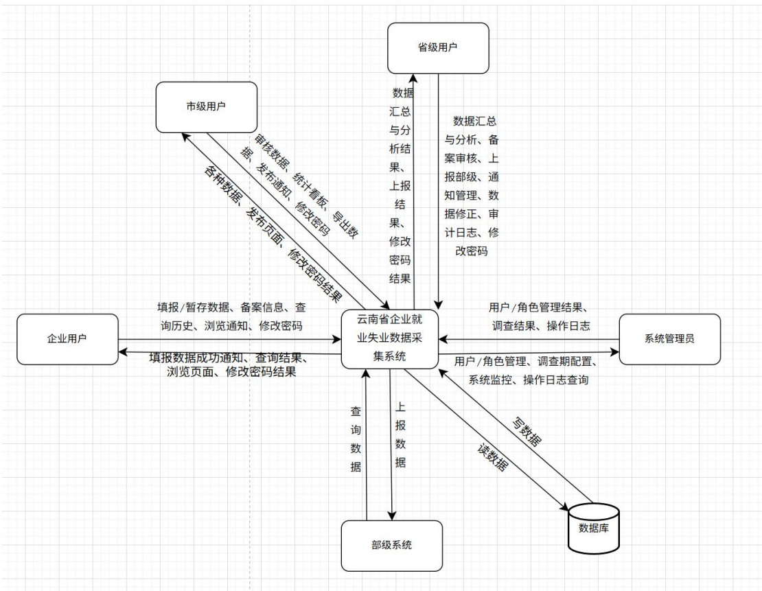
B-5-1 上下文图
