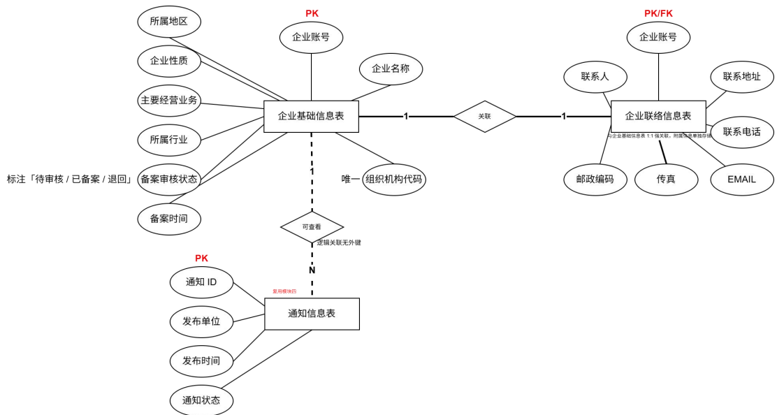
图 B-1-1 企业端：数据采集与备案子系统的 E-R 图
