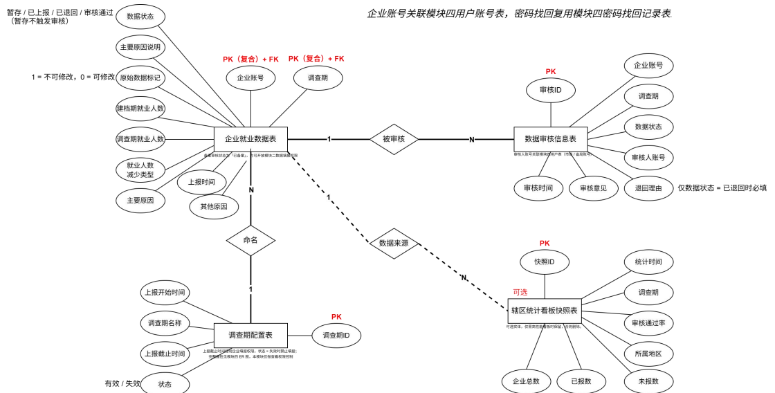
图 B-1-2 市级端：数据审核与辖区调度子系统的 E-R 图
