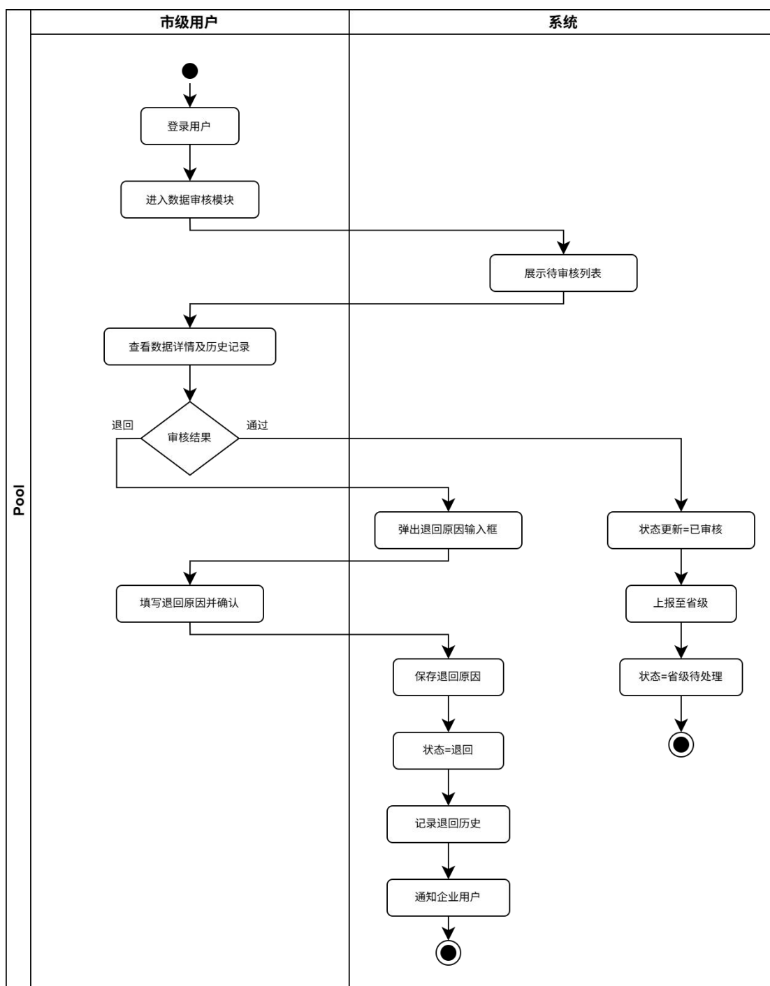
图 B-2-3 市级端数据审核与处理活动图
