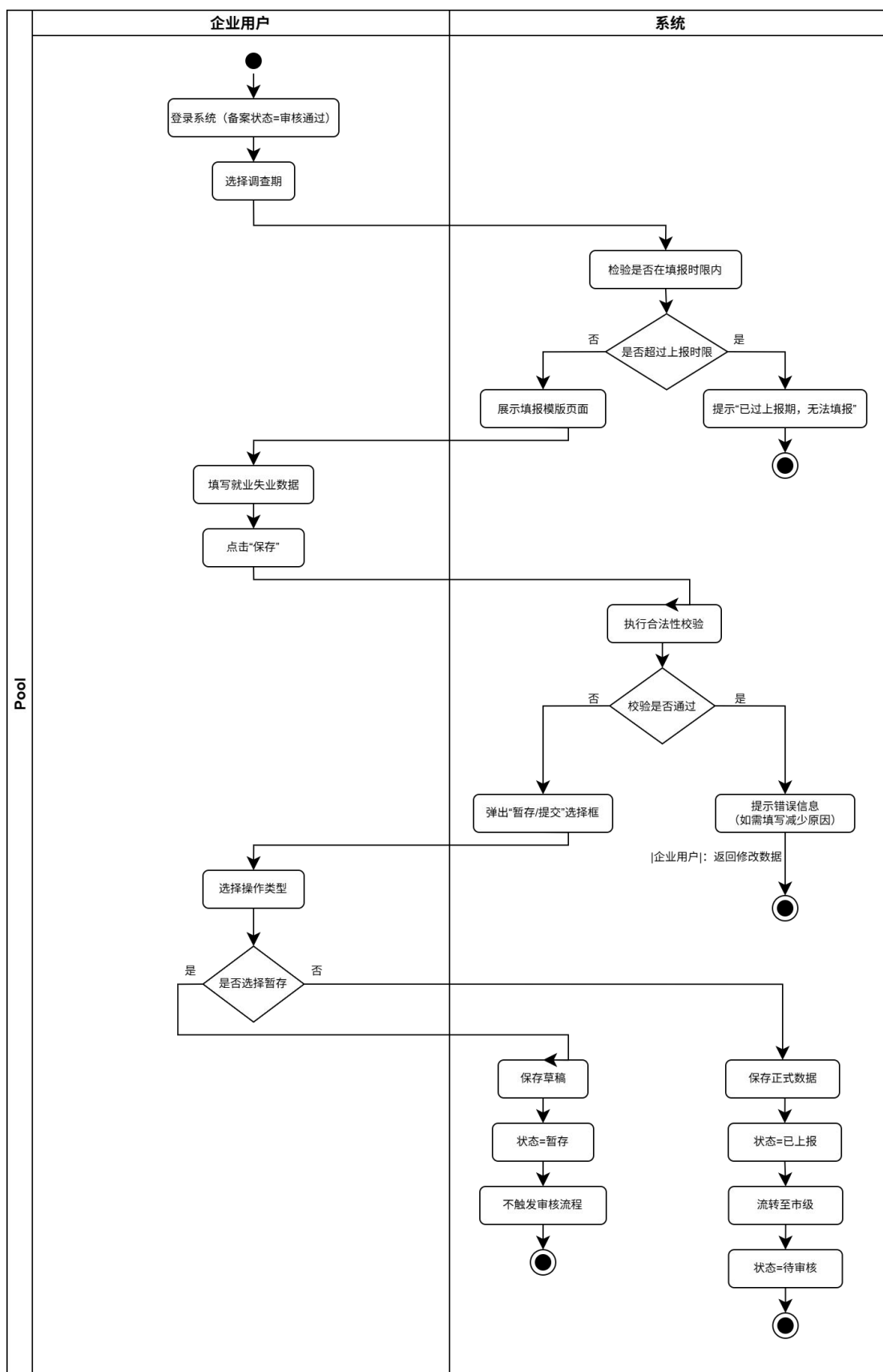
图 B-2-1 企业月度数据填报活动图
