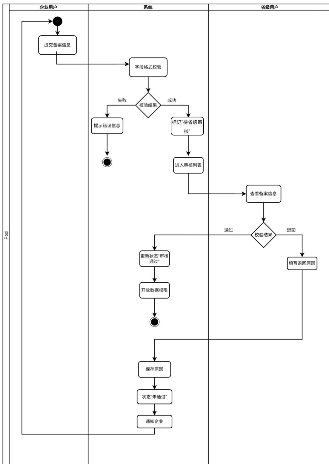
图 B-2-2 企业信息备案与省级审核活动图
