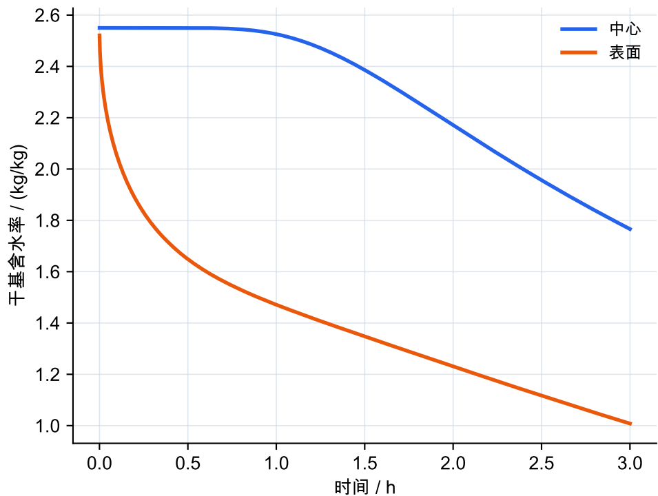
问题2：中心与表面含水率
