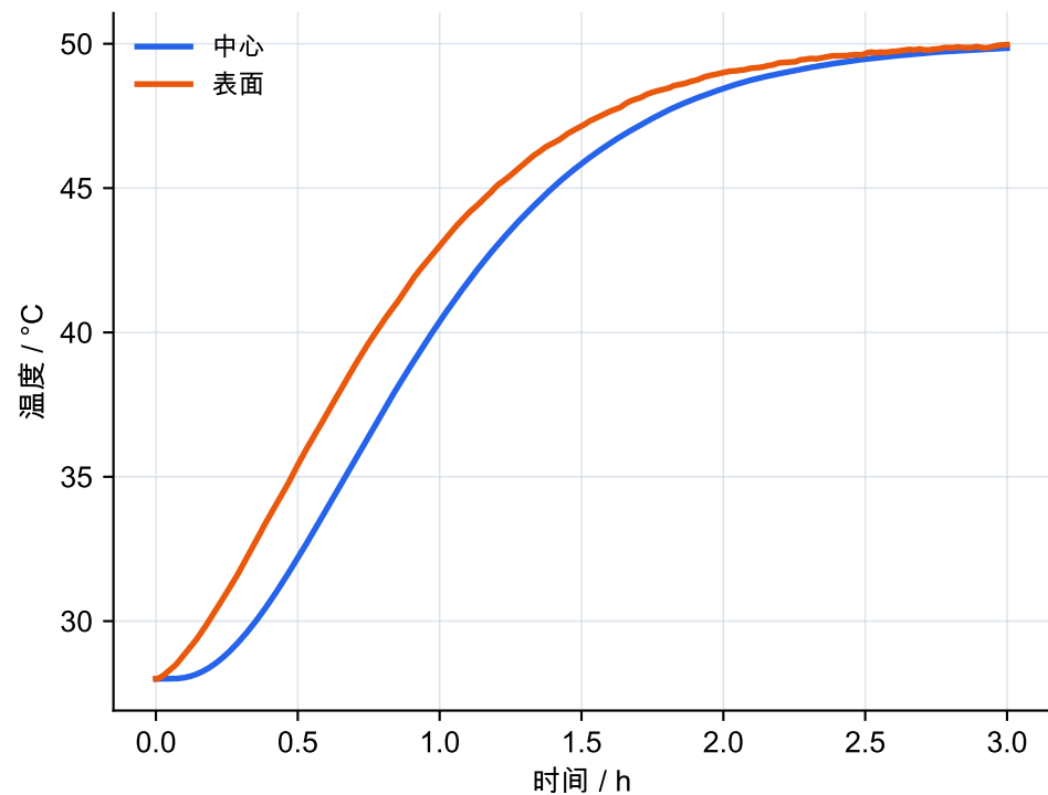
问题2：中心与表面温度
