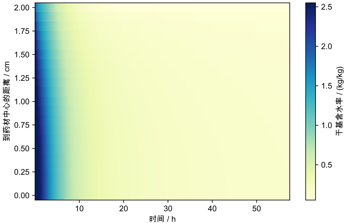
问题3：全过程含水率时空分布
