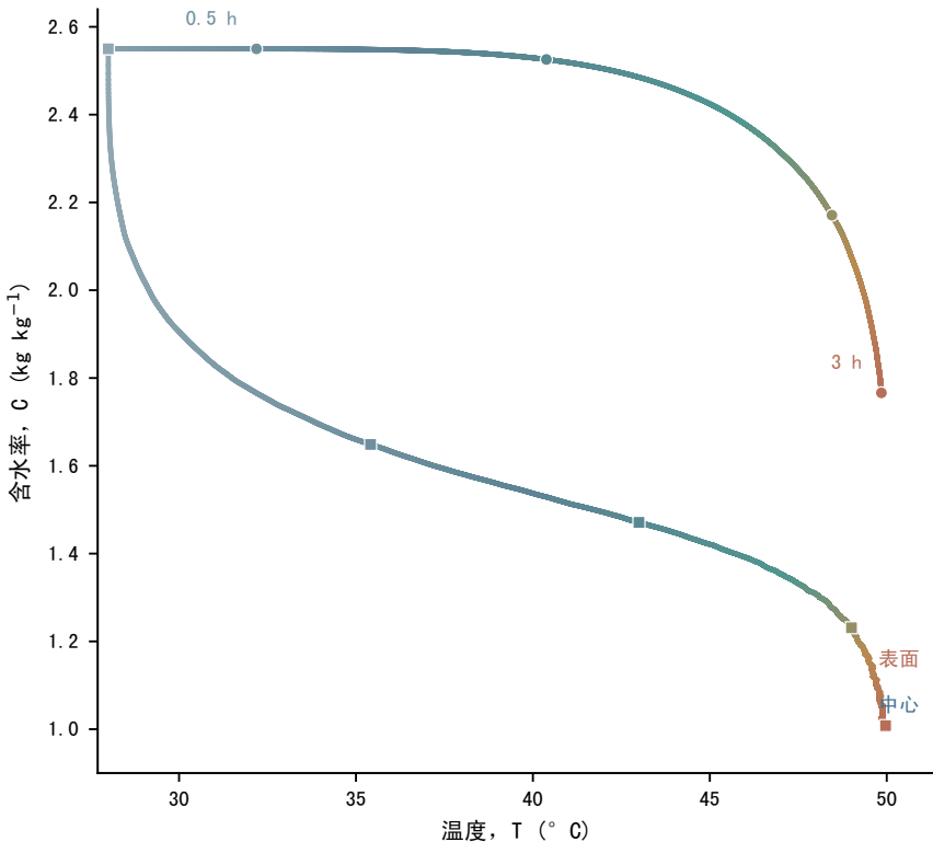
温度 - 含水率状态轨迹
