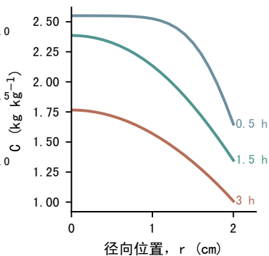
c 含水率剖面
