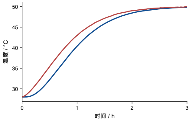
问题2：中心与表面温度
