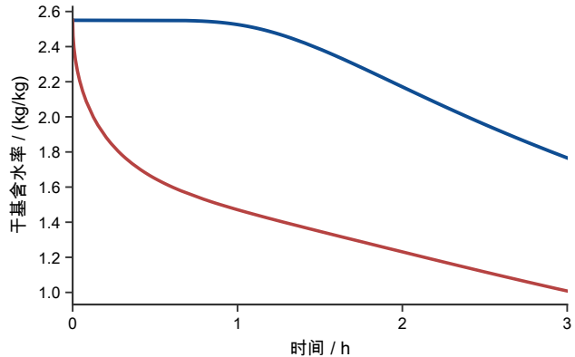
问题2：中心与表面含水率
