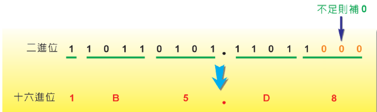
圖 2-11 110110101.11011_2 的十六進位表示法為 1B5.D8_{16}
