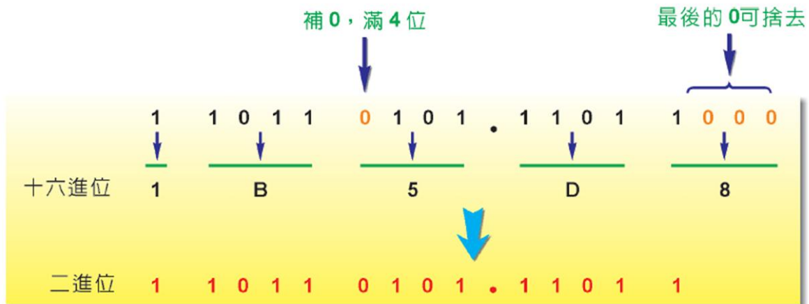
圖 2-12 1B5.D8_{16} 的二進位表示法為 110110101.11011_2
