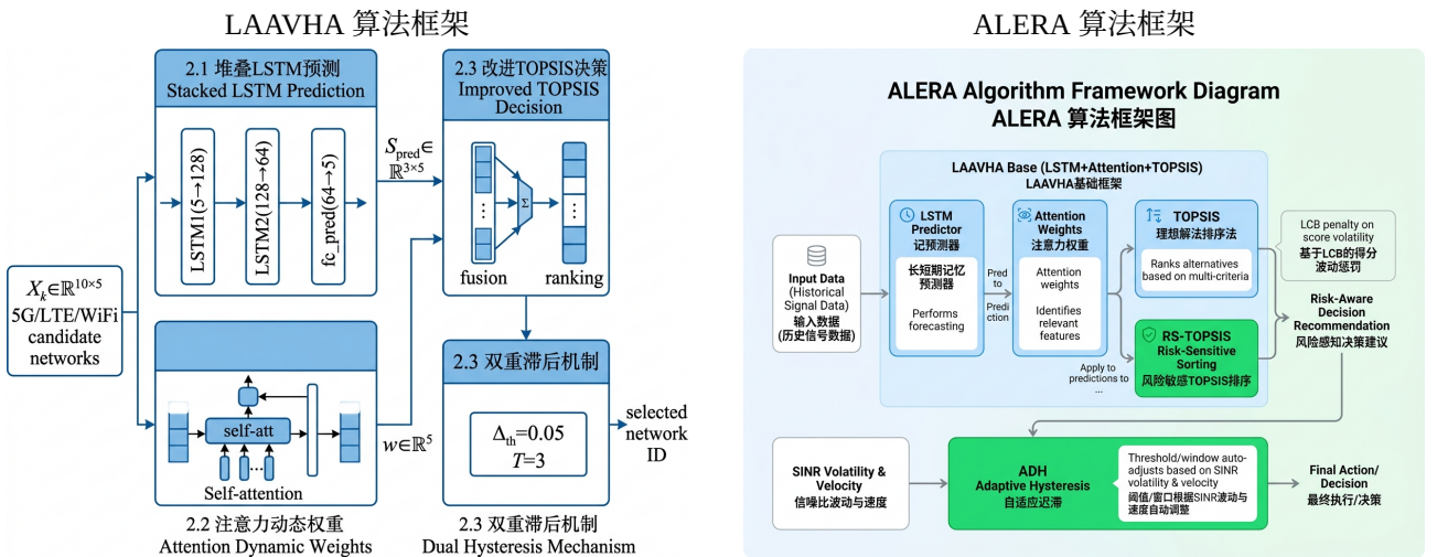
图 2 LAAVHA 与 ALERA 算法框架
