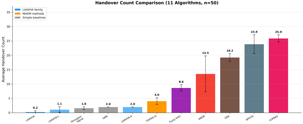
图 4 11 种算法平均切换次数对比 (mean \pm std, n=50)
