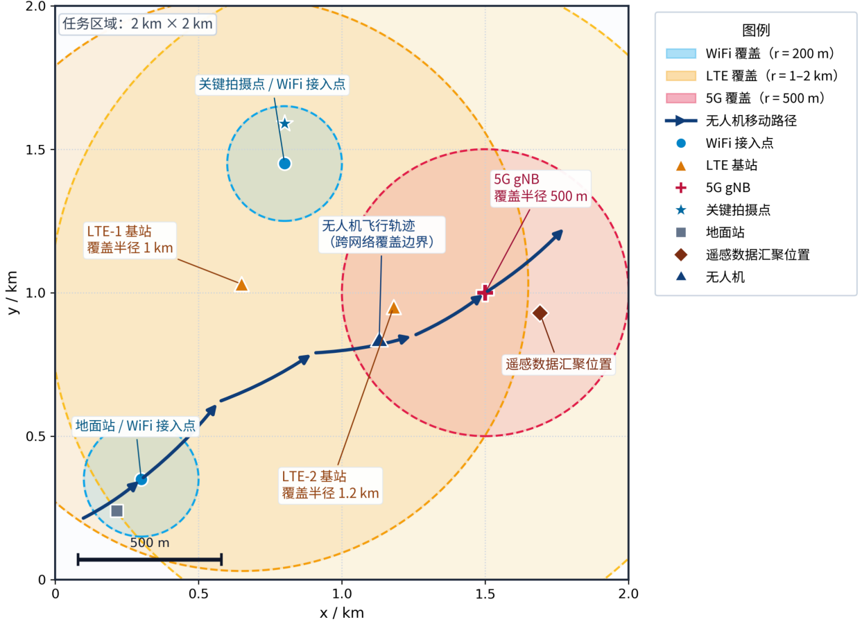
图 1 无人机遥感任务区域中的异构网络覆盖与移动轨迹示意
