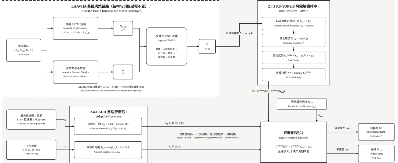
(b) ALERA 算法框架
