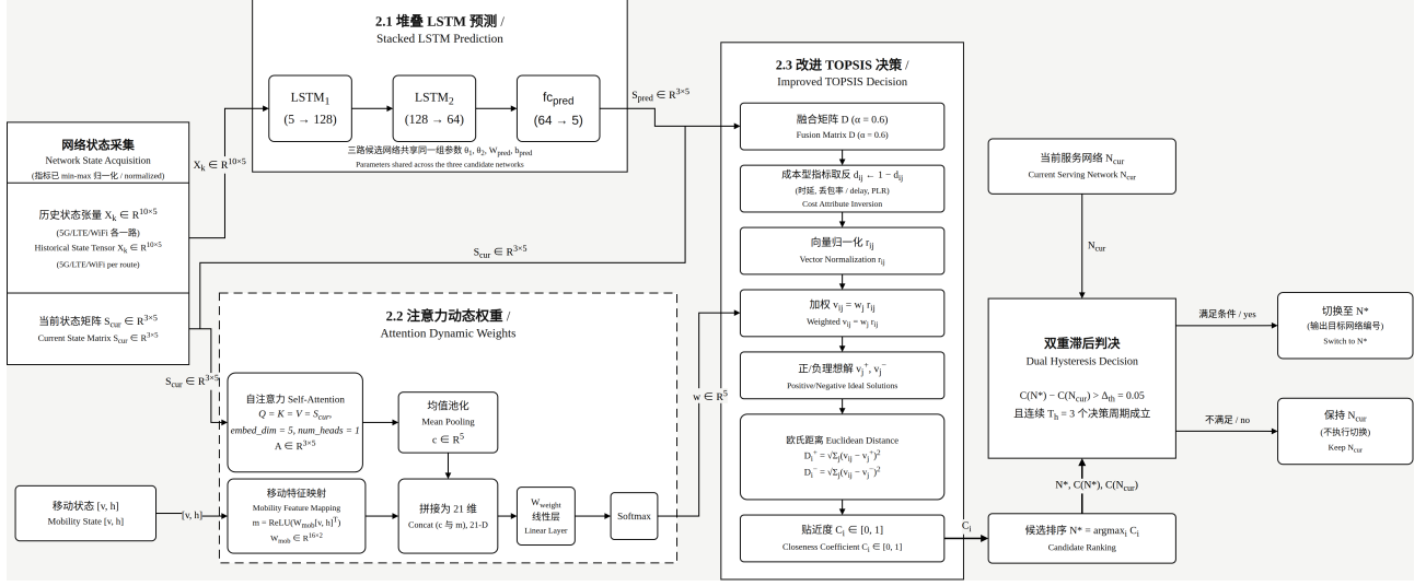
(a) LAAVHA 算法框架
