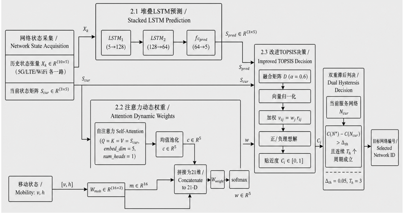
(a) LAAVHA 算法框架
