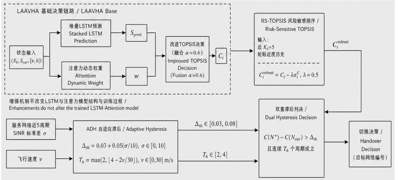
(b) ALERA 算法框架
