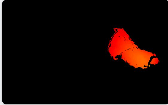
같은 순간의 depth 맵 — 유효범위(~0.72m) 안의 팔·몸통만 색이 채워지고, 그보다 먼 나머지 전부는 무효(검정)
