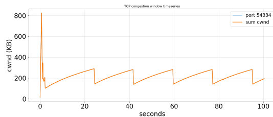
CWND ( q=20 ) - without AQM
