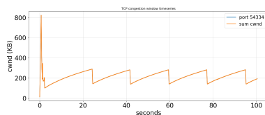
CWND (q=100)
