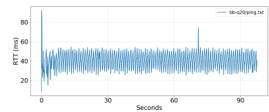
RTT (q=20)
