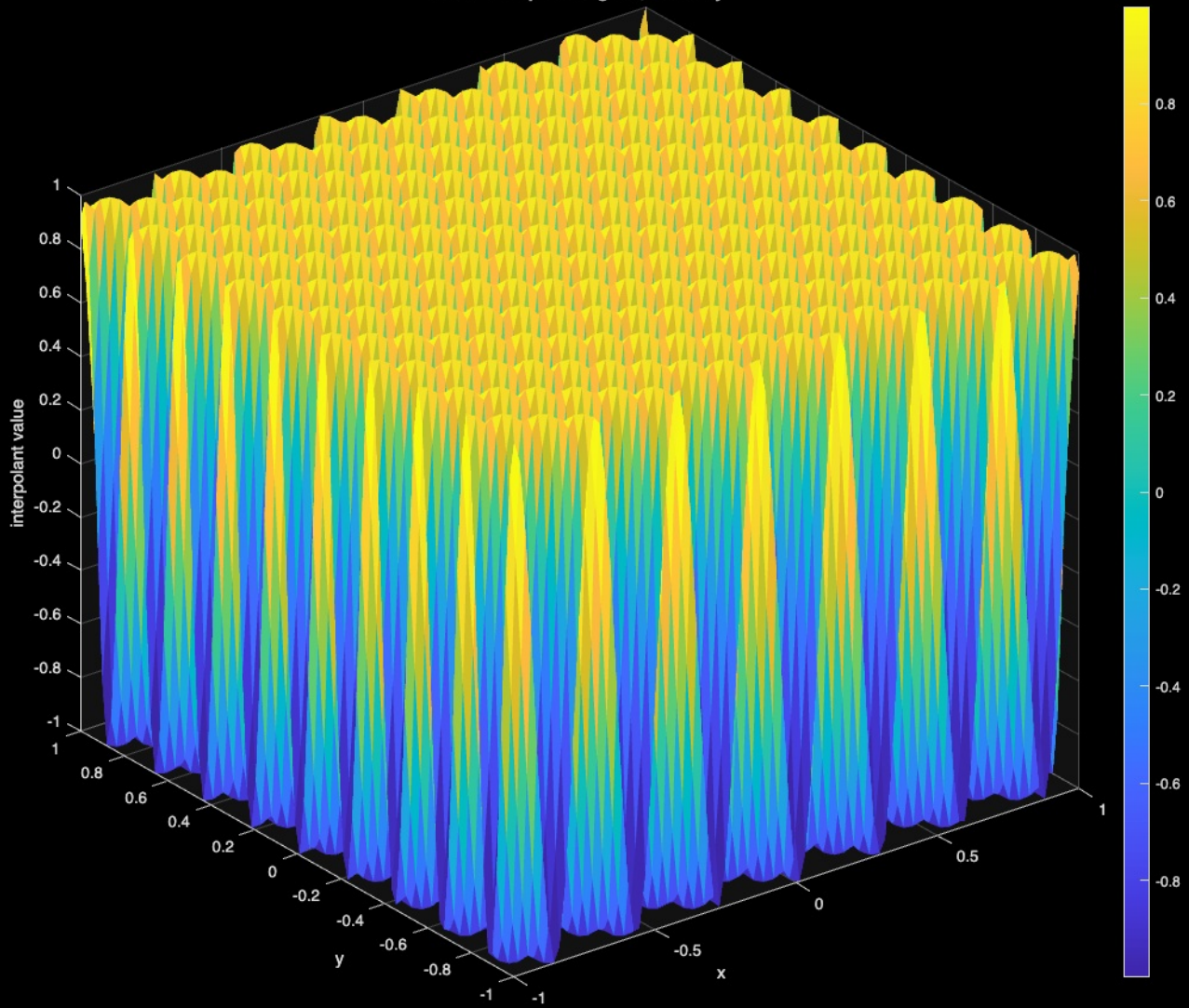
EFTT interpolant: \text{genz}_{\text{oscillatory}}
