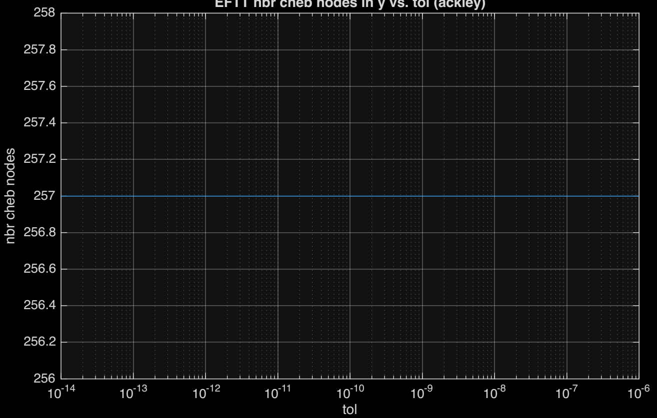
EFTT nbr cheb nodes in y vs. tol (ackley)
