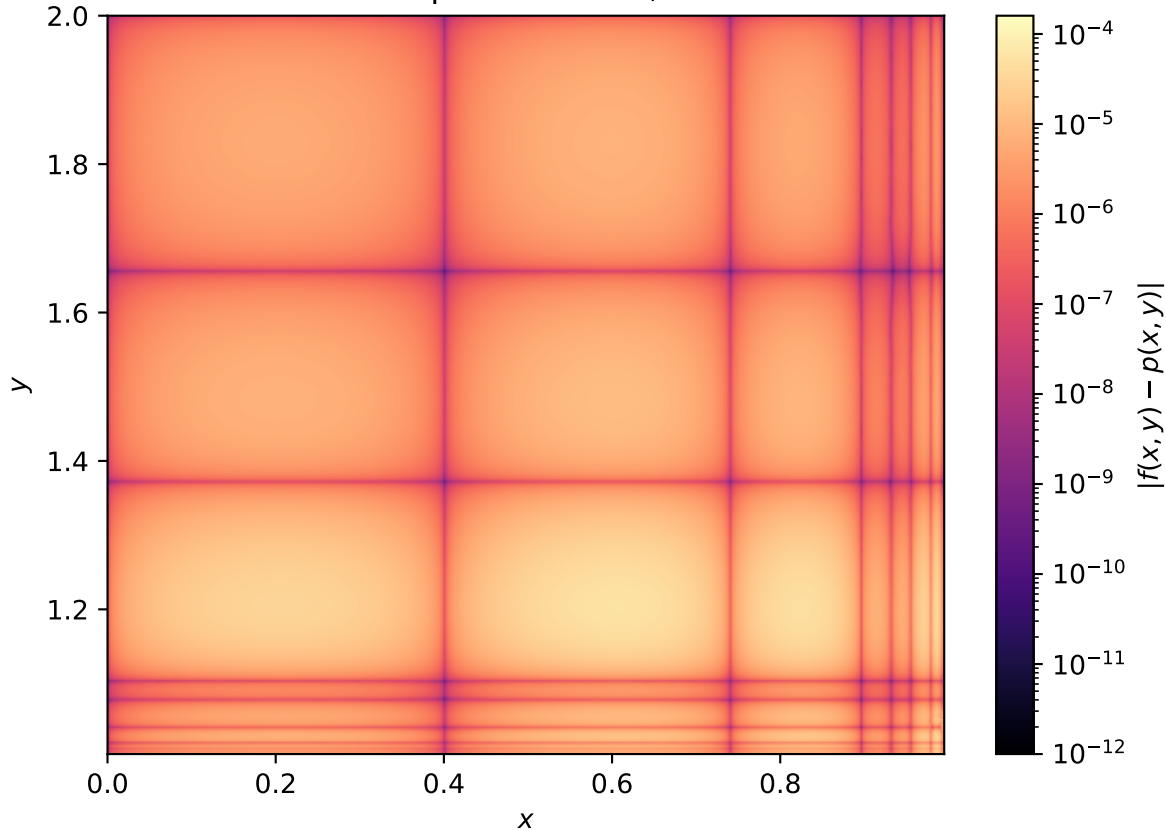
Absolute interpolation error, s = 1e - 02
