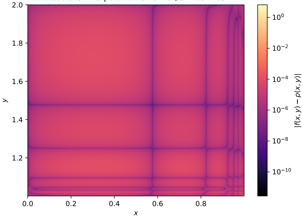
Absolute interpolation error for, s = 1e - 03
