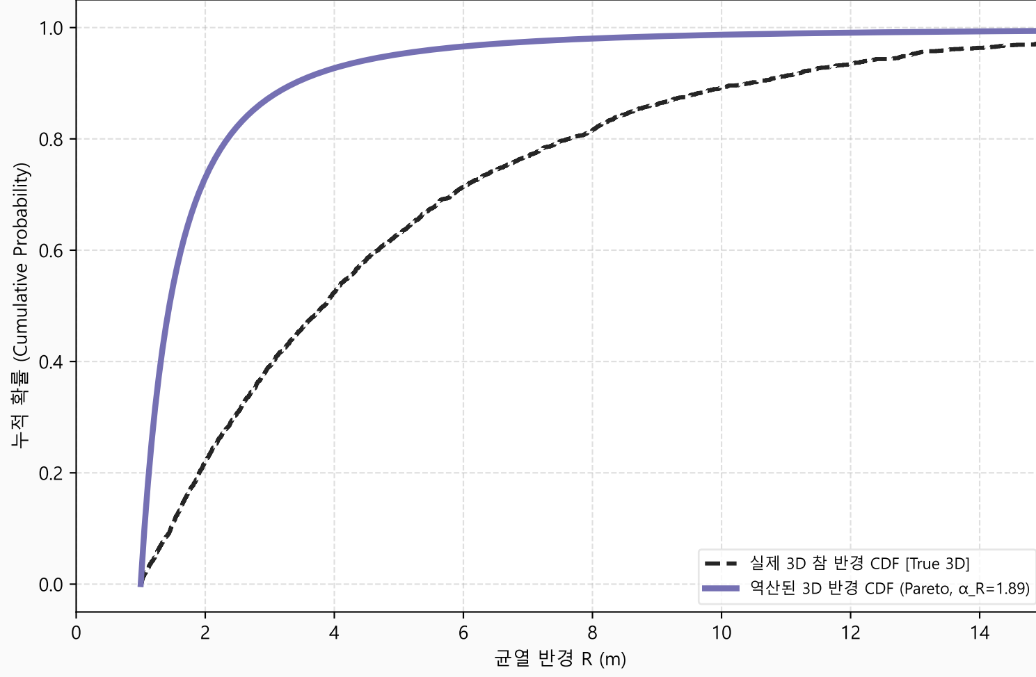
균열 세트 5 - 3D 참 반경 누적분포 (CDF) 역산
