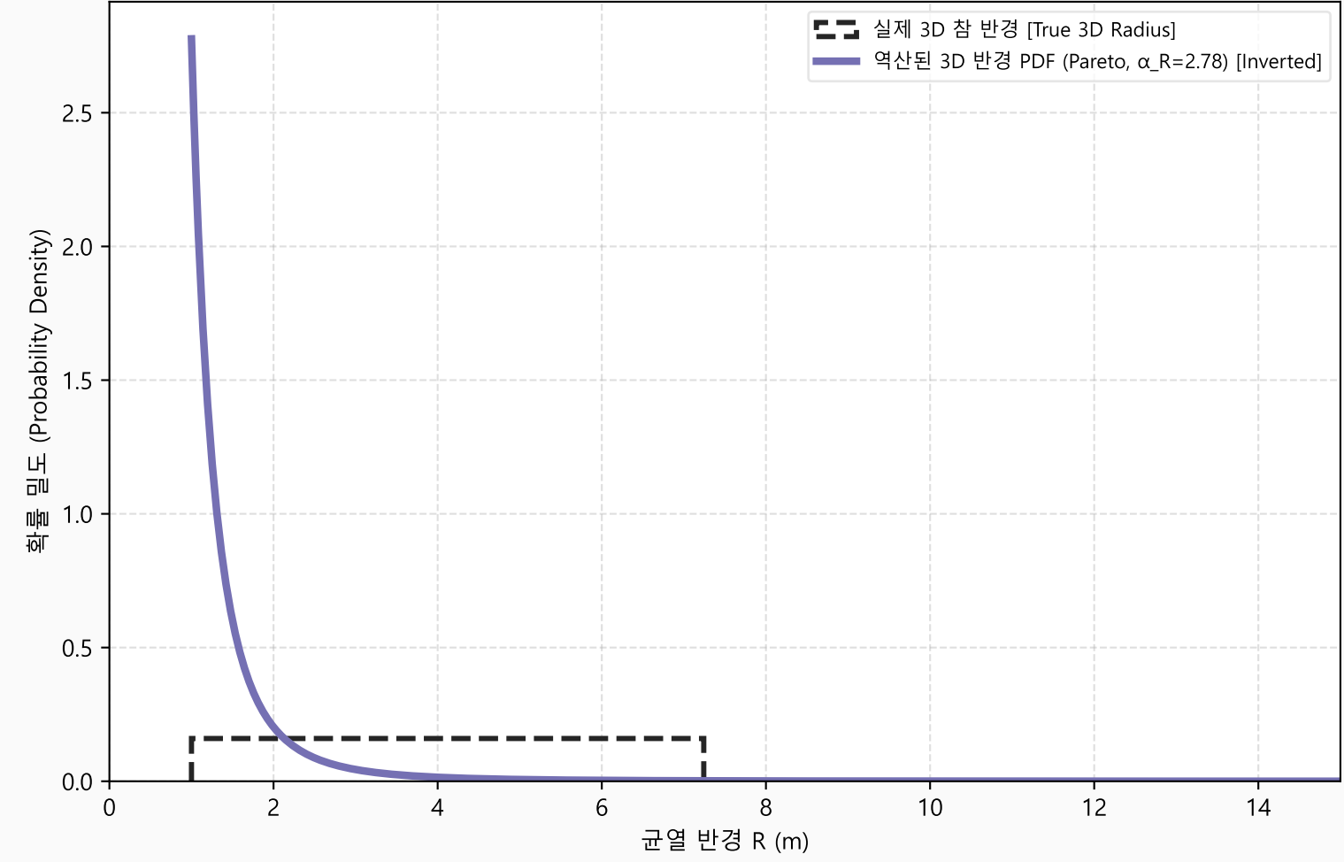
균열 세트 3 - 3D 참 반경 분포 역산
