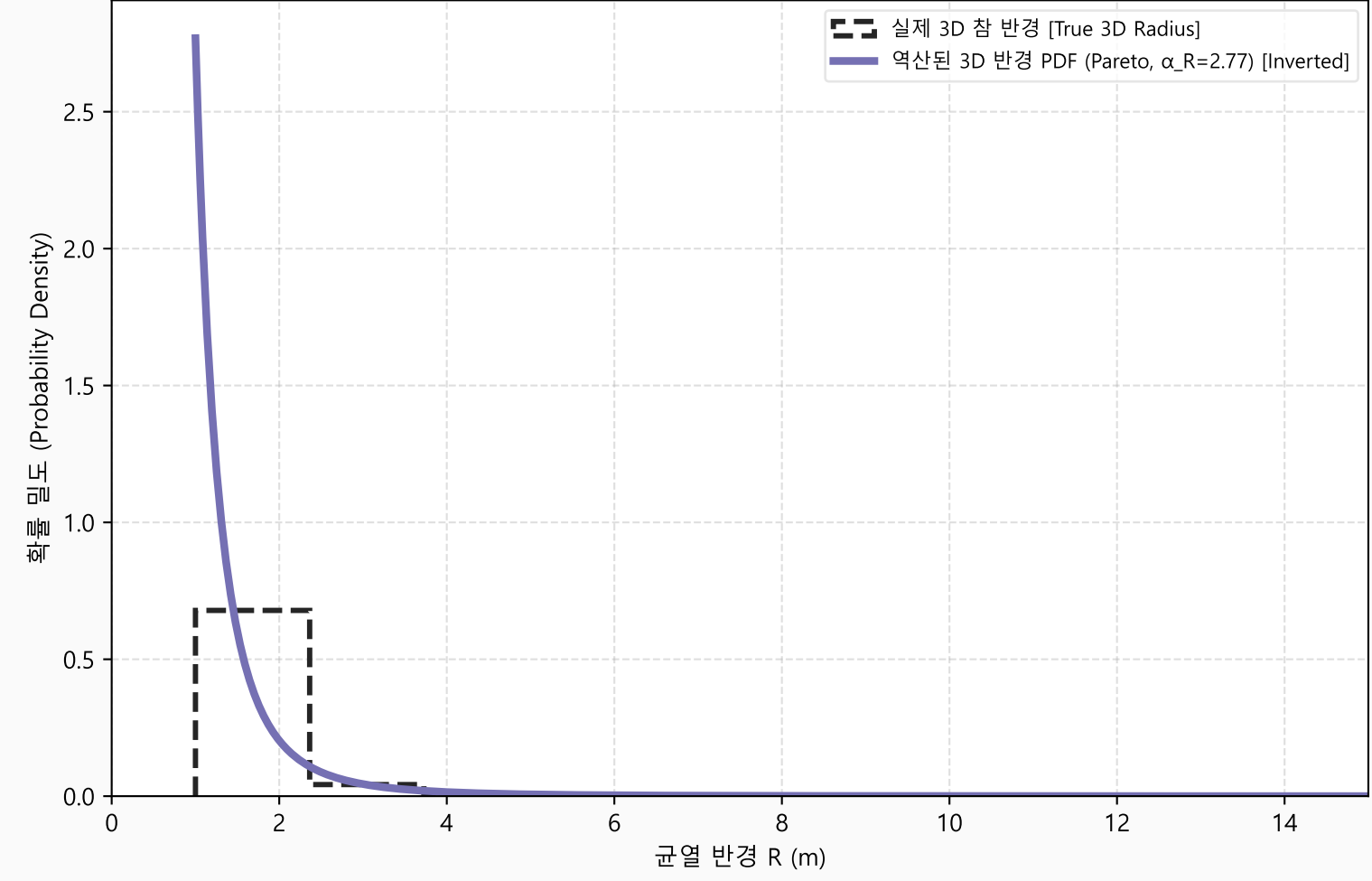
균열 세트 4 - 3D 참 반경 분포 역산
