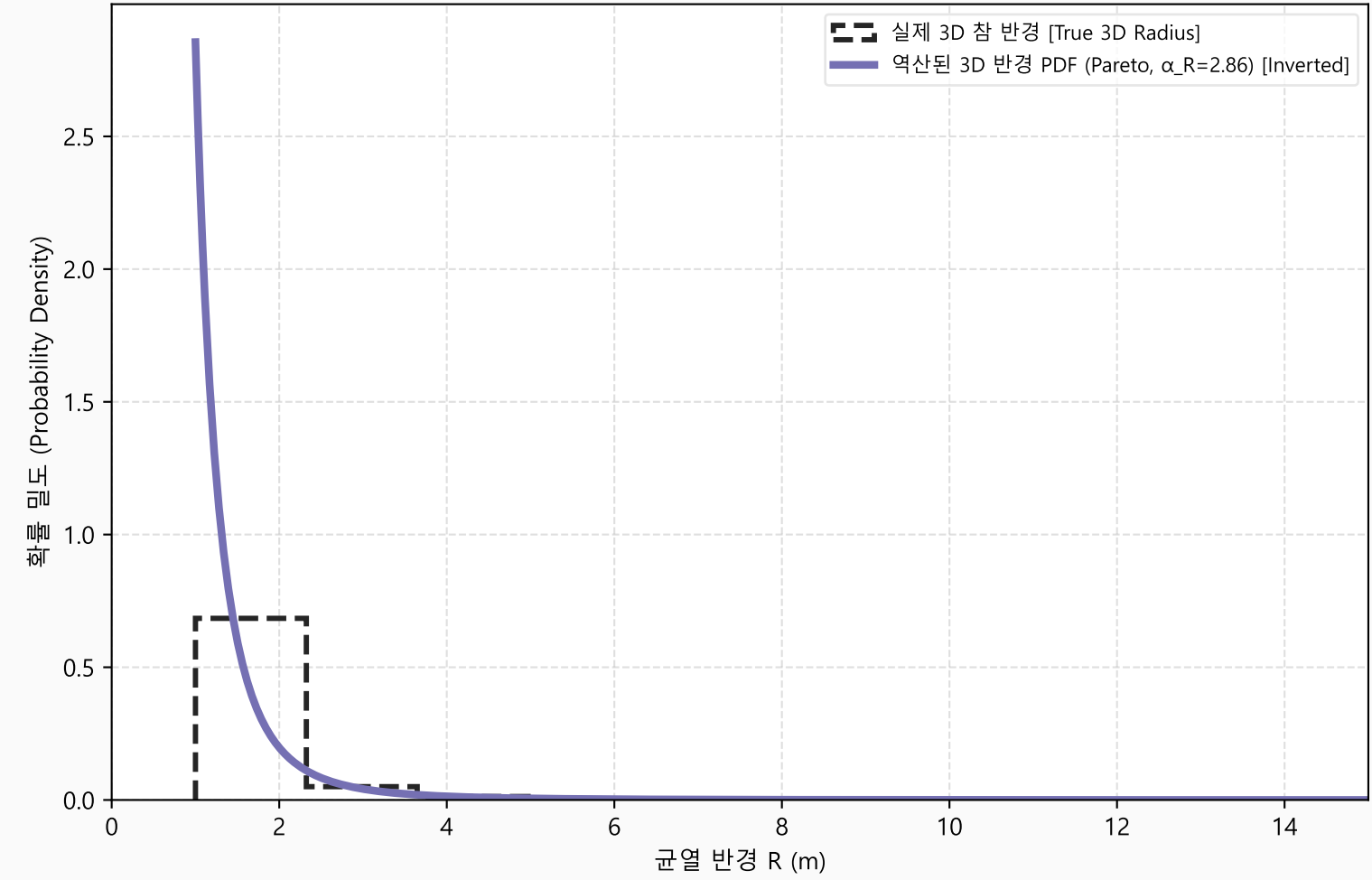
균열 세트 2 - 3D 참 반경 분포 역산
