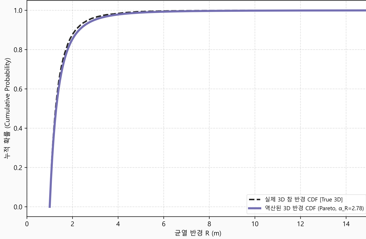
균열 세트 3 - 3D 참 반경 누적분포 (CDF) 역산
