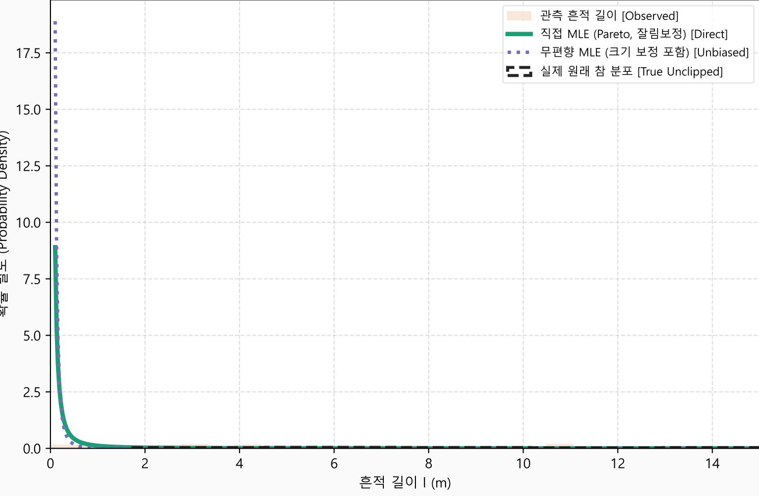
균열 세트 5 - 확률밀도함수 (PDF) 비교
