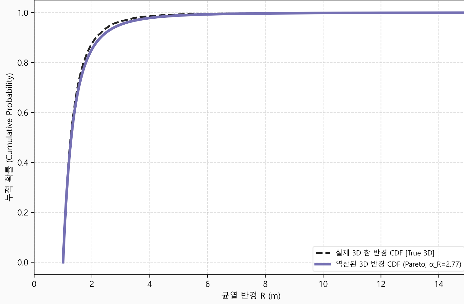
균열 세트 4 - 3D 참 반경 누적분포 (CDF) 역산
