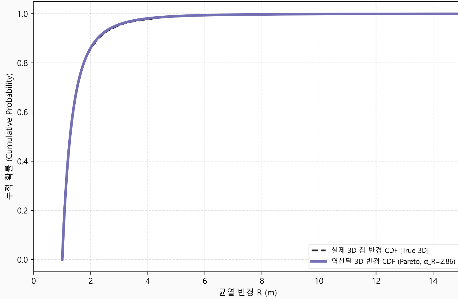
균열 세트 2 - 3D 참 반경 누적분포 (CDF) 역산
