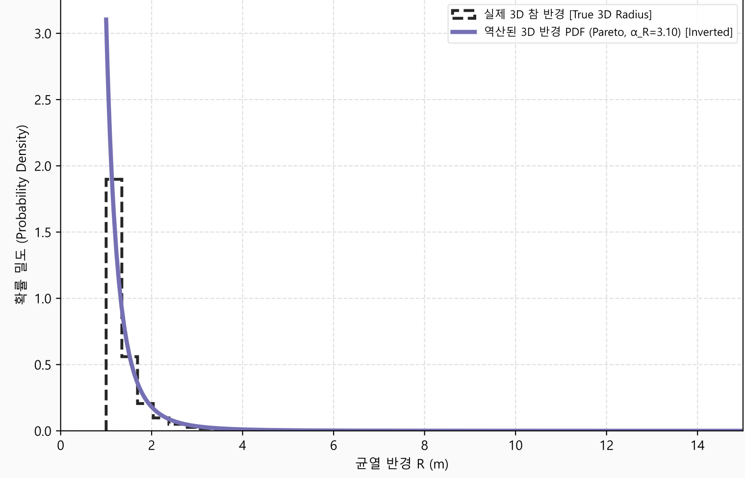
균열 세트 5 - 3D 참 반경 분포 역산
