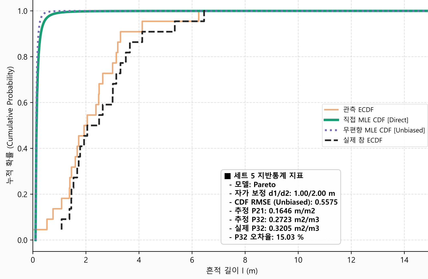
균열 세트 5 - 누적분포함수 (CDF) 비교
