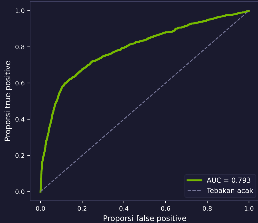
Kurva ROC
