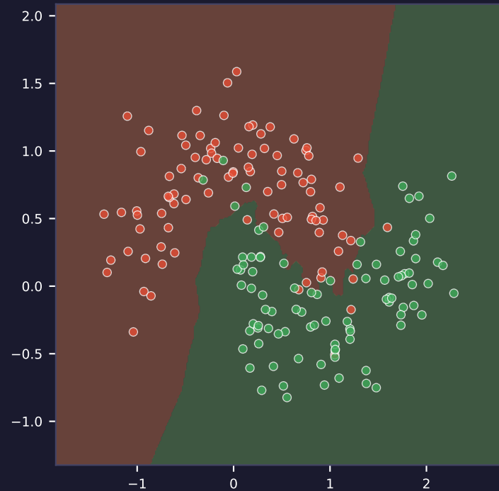
KNN (K=5) Acc=0.972
