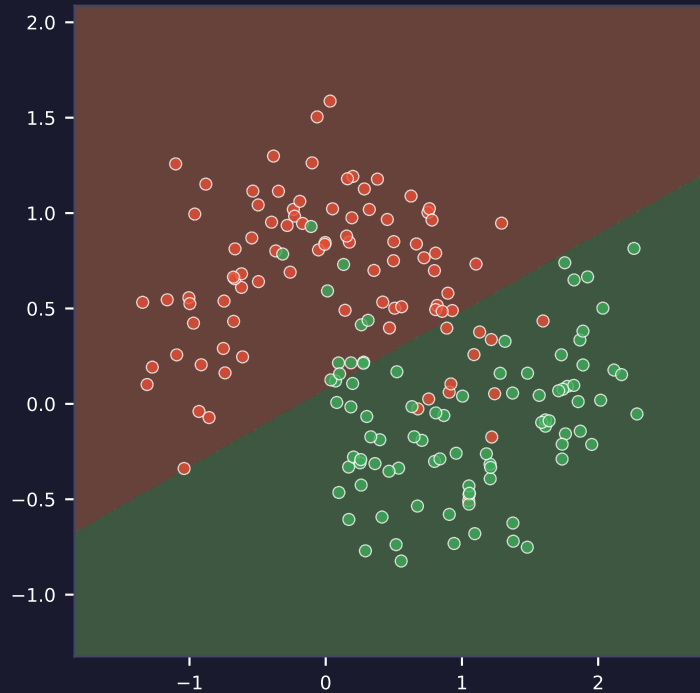
SVM Linear Acc=0.944
