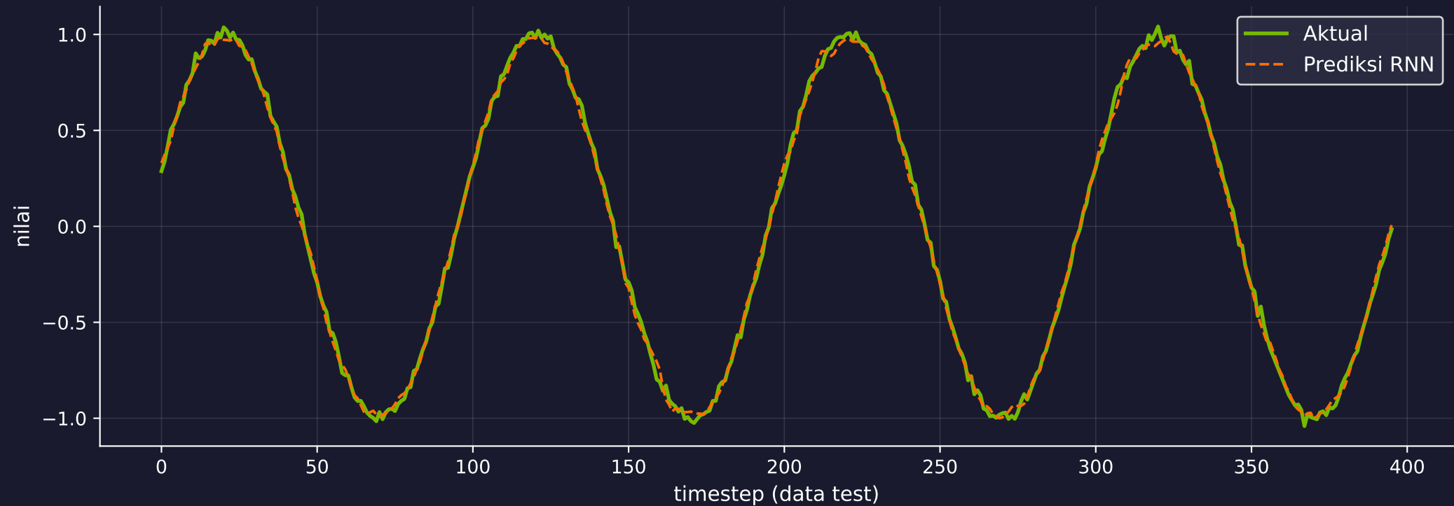
Prediksi Gelombang Sinus dengan SimpleRNN(32) — MAE = 0.0246
