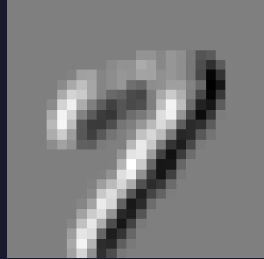
Hasil konvolusi
