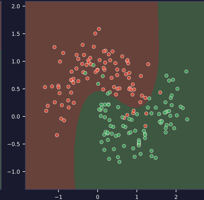
SVM RBF Akurasi = 0.972
