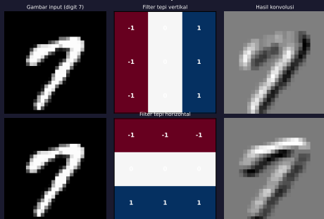
Konvolusi manual: filter tepi vertikal vs horizontal
