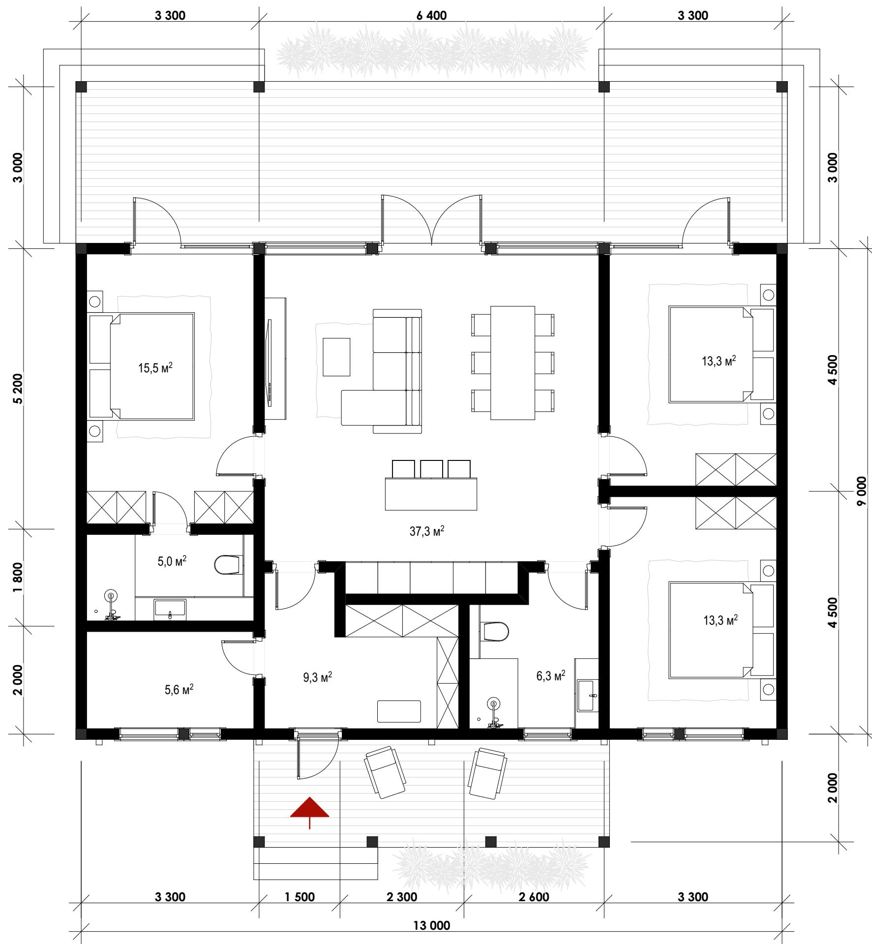
ПЛАН шале 4 (13x9)
