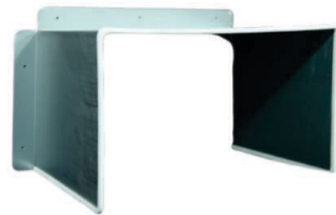
빗물커버 (철제/0.3T)
