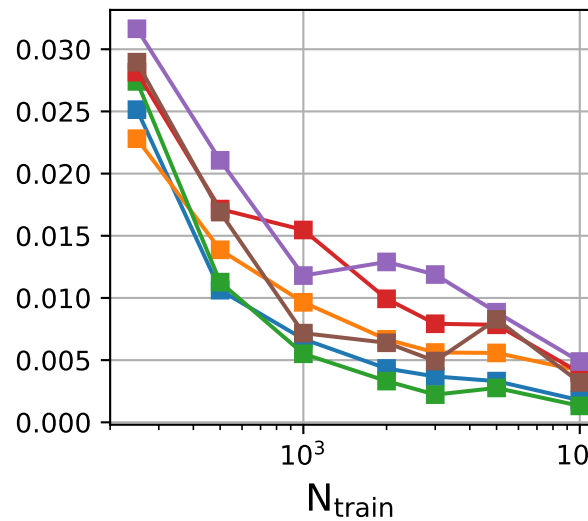
KL-div tails
