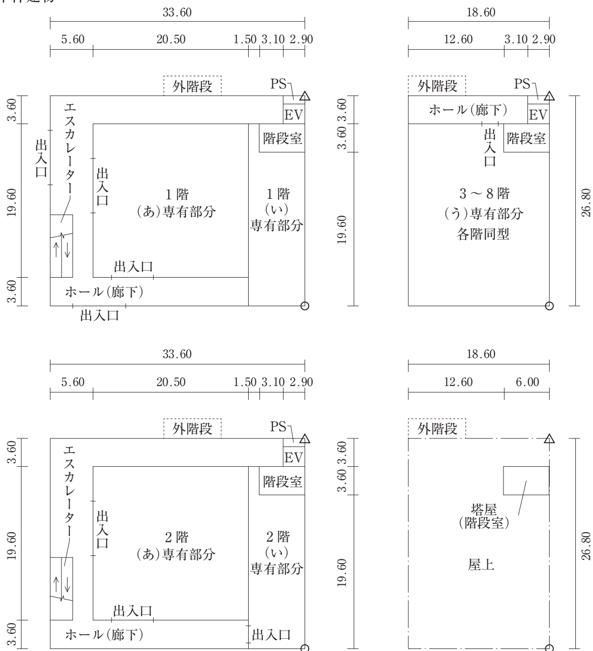
図3・平面図
