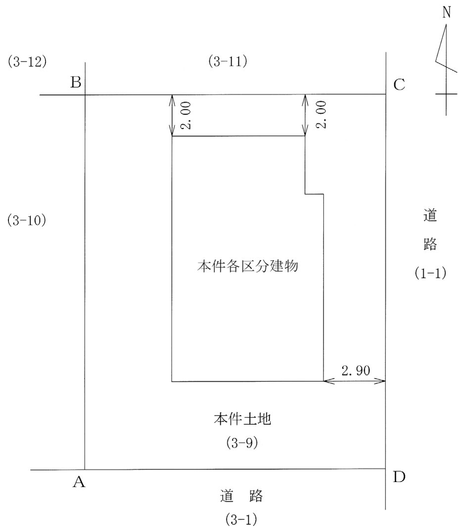
図1〔建物配置図〕
