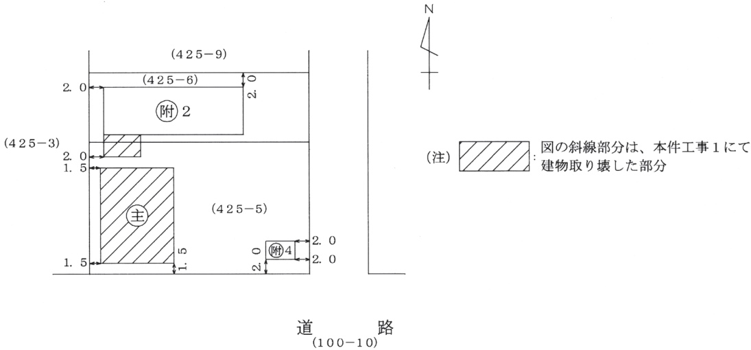
(本件工事 1 一敷地図・建物配置図 1)
