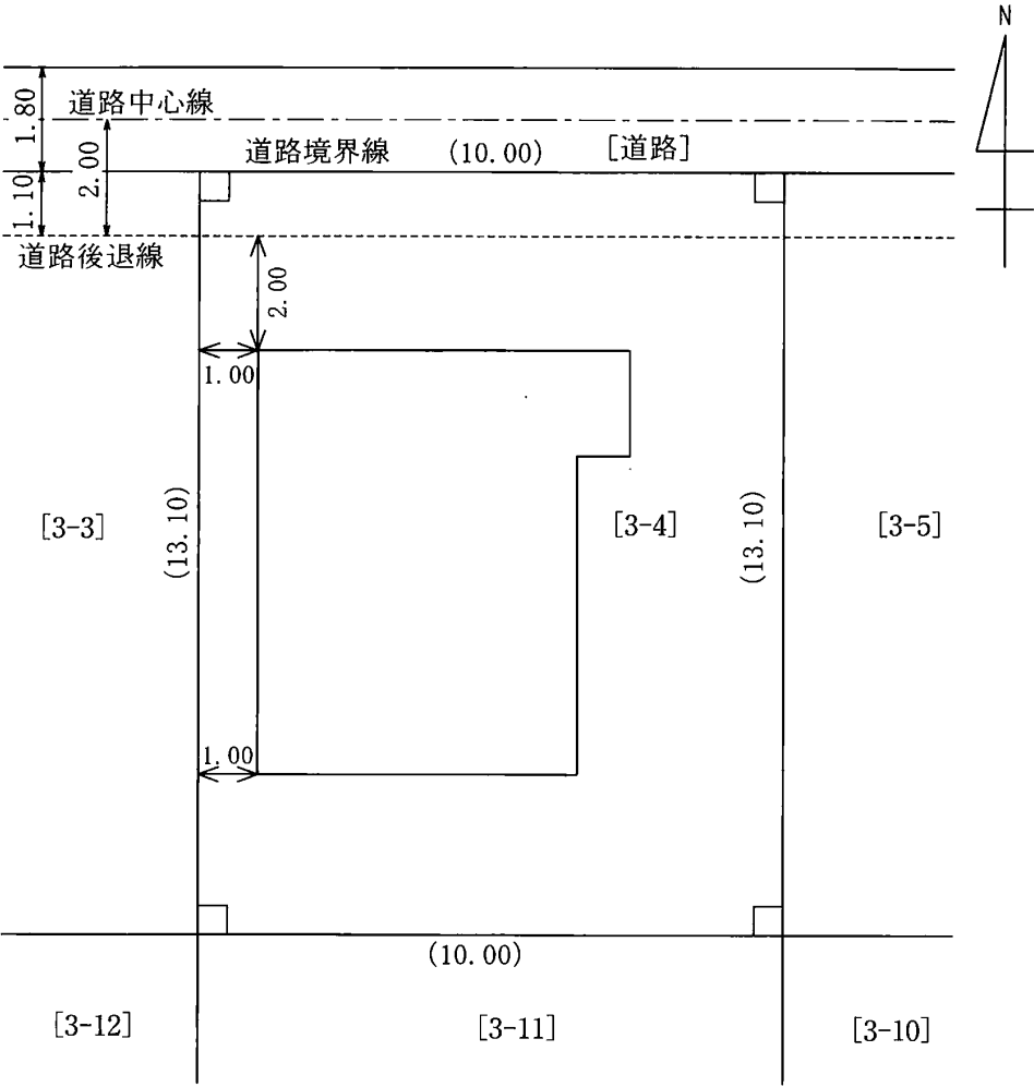
〔配置図〕
