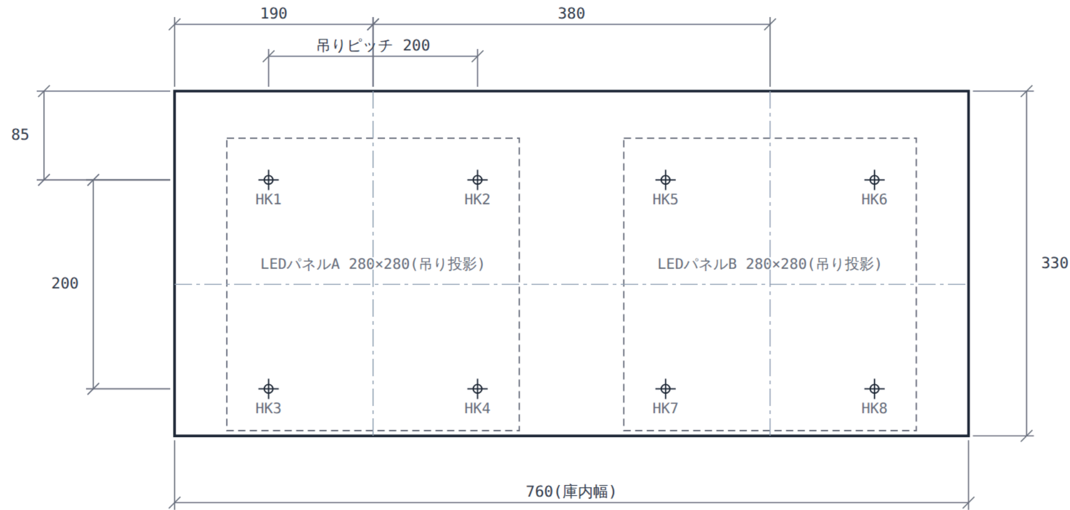
天井伏図(下から見上げ・Y=0が背面)
