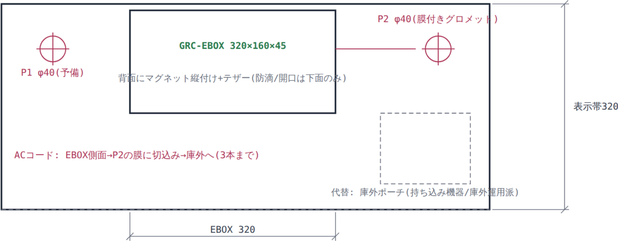
背面上部の電源ボックスとAC引き出し (背面を透過表示・Z=700~1020)
