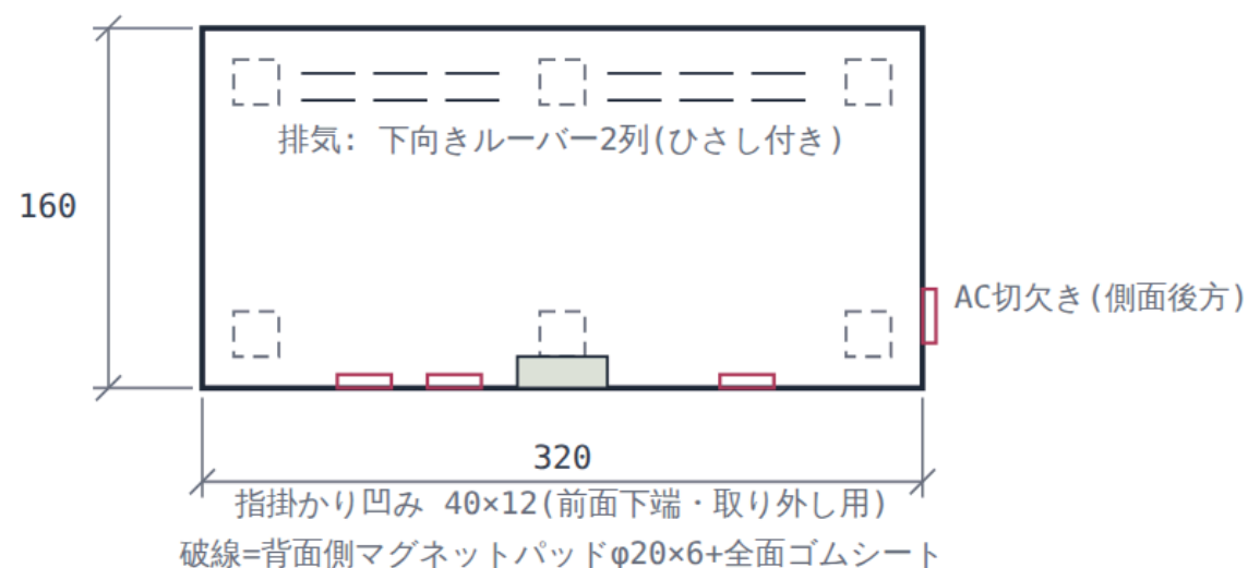
正面図(壁付け姿勢・扉側から見える面)
