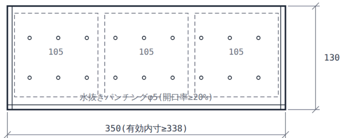
平面図(3鉢配置)
