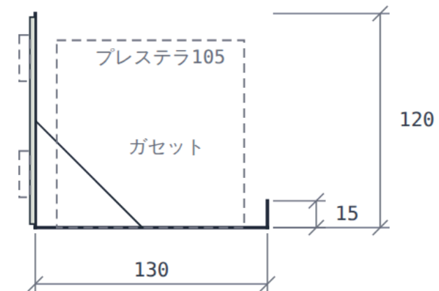
側面図
