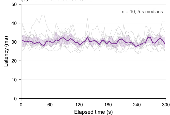
(d) PC–VR shared-state RTT
