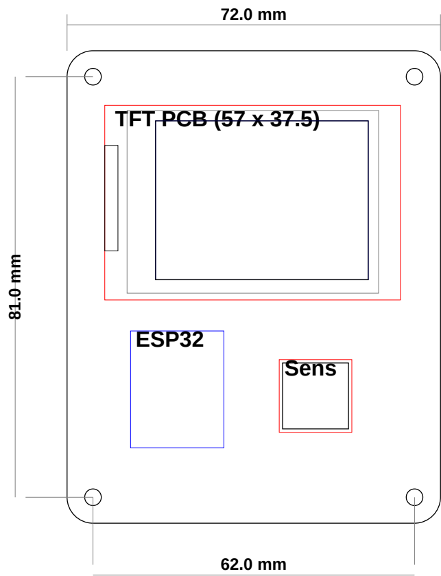
Vista 2: Acrílico Frontal Transparente sobre Componentes (Escala 1:1)
