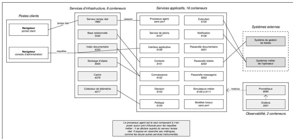
FIGURE 4.5 – DIAGRAMME DE DÉPLOIEMENT DE LA PLATEFORME
